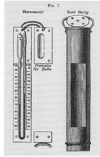
"Miller-Casella" deep-sea thermometer. "ミラー・カッセラ" 深海用温度計
