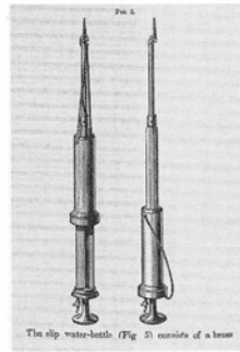
Slip water-bottle. スリップ式採水器
