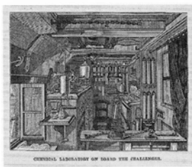
Chemical laboratory on board the Challenger. チャレンジャー号船内の化学実験室
