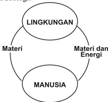
Gambar 1.2. Hubungan antara manusia dan lingkungan dengan aliran materi, energi, dan informasi
