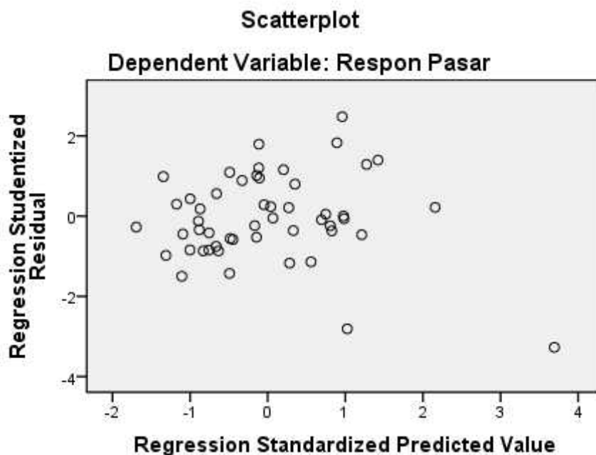
Gambar 4.3 Uji Heteroskedastisitas
