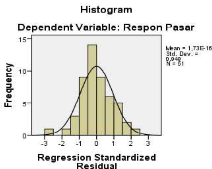
Gambar 4.1 Grafik Histogram
