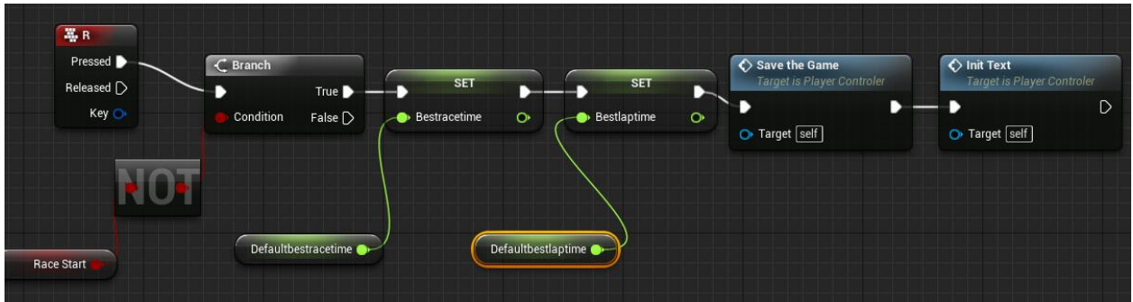
Slika 9.26 Skripta pritiska tipke R
