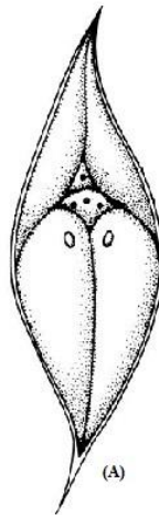
Slika 10. Lepidodendron - rekonstrukcija (A) i fosilni ostaci (B) baze lista. Mjerilo = 3.5 mm. (preuzeto i prilagođeno s Taylor, Taylor i Krings, 2009.)
