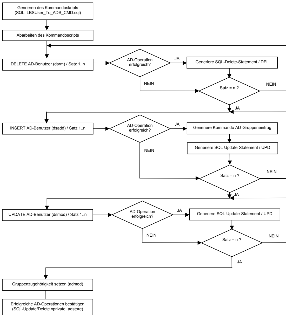
Abb. 5: Schematische Darstellung der Bearbeitung auf dem AD-Client.
