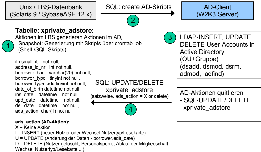
Abb. 3: Abgleich zwischen LBS-Datenbank und Active Directory.
