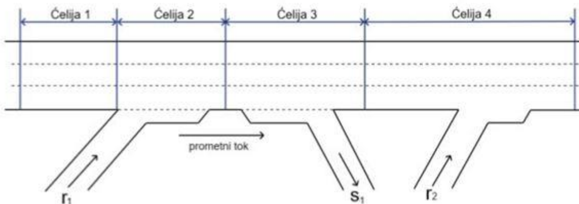
Slika 11. Raspored ćelija [22]
