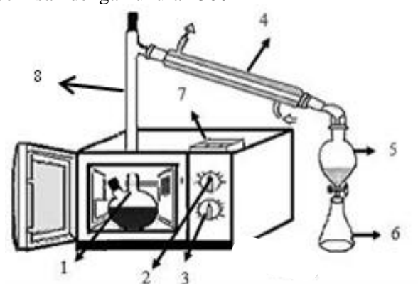
Gambar 1 Seperangkat hydro distilation microwave
