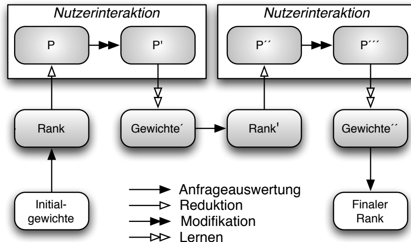
Abbildung 1: Verfeinerung von Gewichten durch Nutzerinteraktion mittels Präferenzen P
