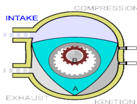
Slika 3 Wankel motor
