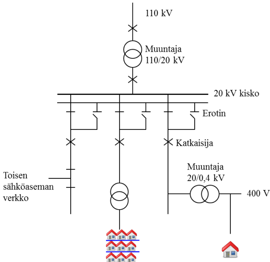
Kuva 2. Sähkönjakeluverkon pääkaavio.
