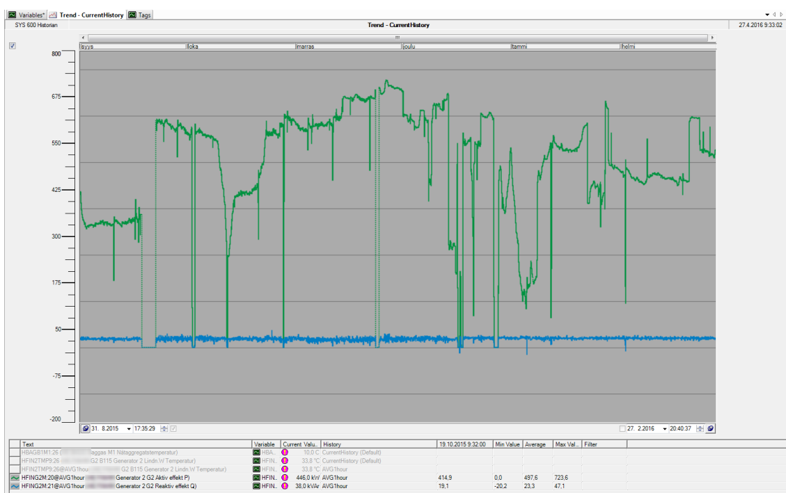
Kuva 10. Kuvaaja-ikkuna, jossa on esitetty pätö- ja loisteho ajan funktiona.
