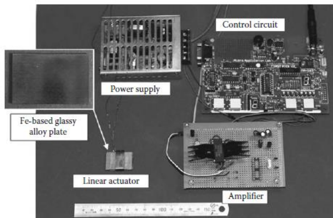
Slika 5.15 Elektronički uređaj na bazi slitina metalnog stakla [2]
