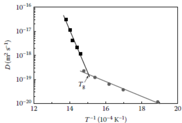
Slika 4.7 Ovisnost difuzije o temperaturi [4]
