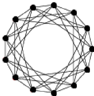
Slika 1.2: Paleyev graf P(13)
