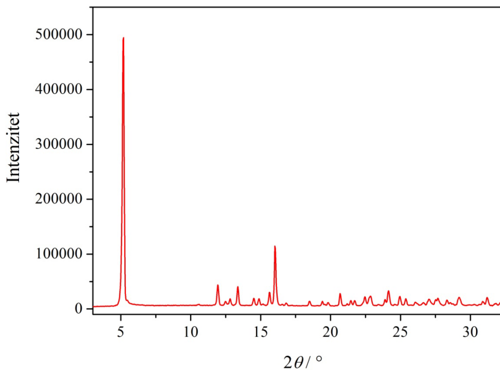
Slika 20. Difraktogram pripravljene soli OMP-K.
