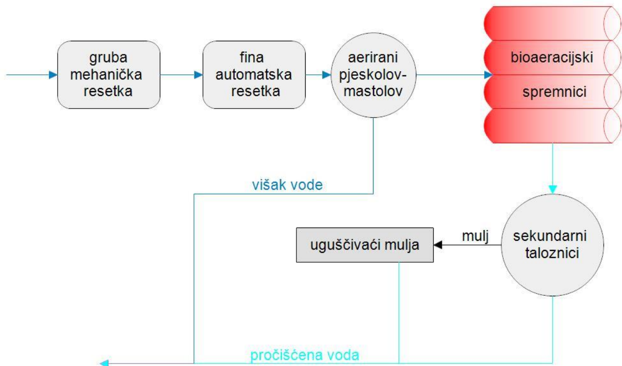
Slika 8. Shematski prikaz sustava za pročišćavanje komunalne otpadne vode
