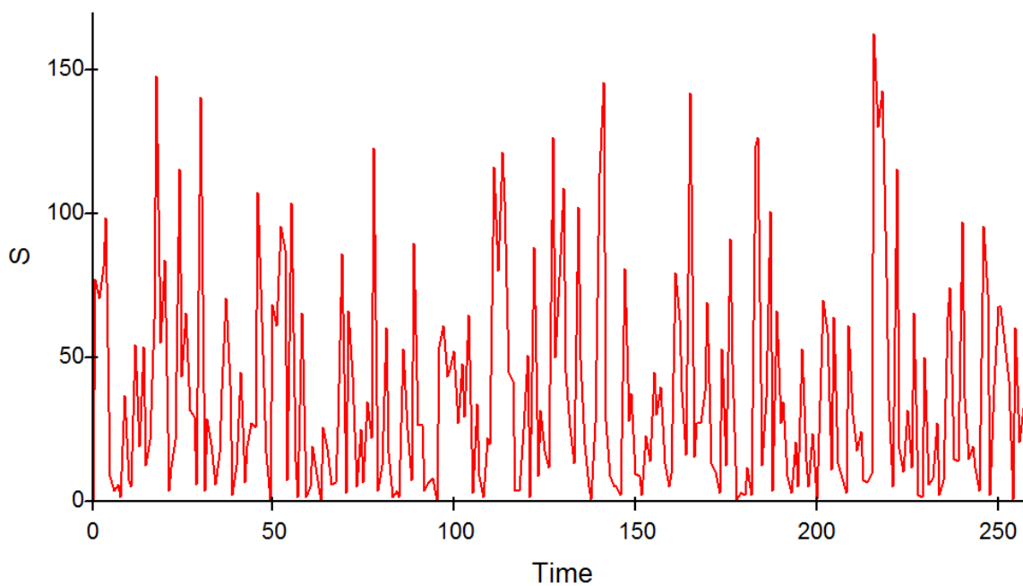
Slika 26. Rezultati simulacije koncentracije organske tvari na izlazu iz bioeracijskog spremnika
