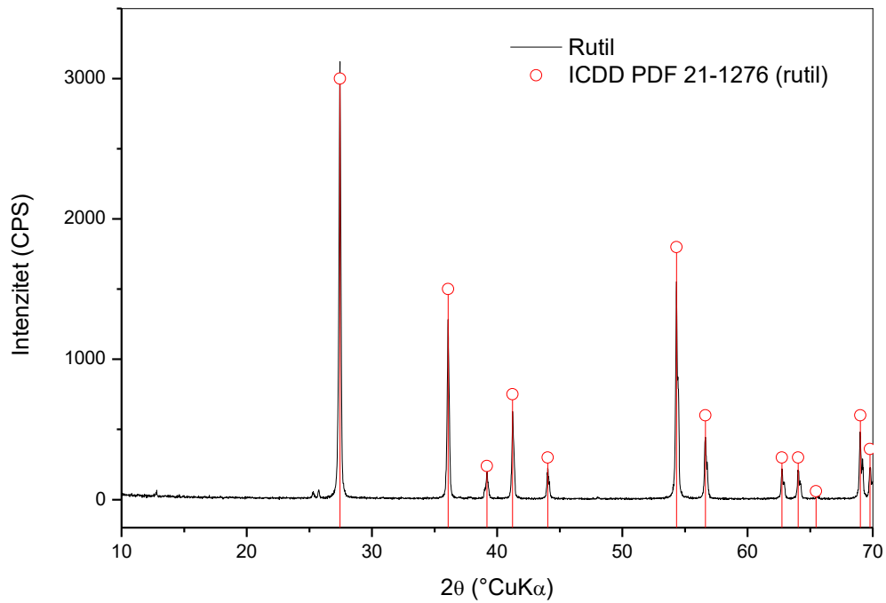
Slika 20. Difraktogram uzorka TiO 2 (Tioxide).
