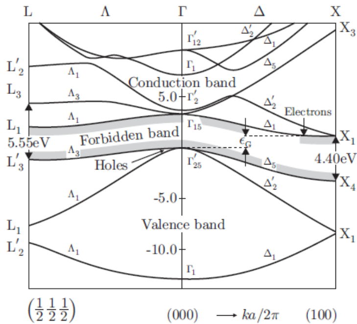
Slika 8. Struktura silicija u smjeru (100) te (111) . Osjenčano područje prikazuje najniži dio (nezaposjednut pri T = 0 K) vodljive vrpce te najvišu dio (zaposjednut pri T=0 K) valentne vrpce sa zabranjenom zonom između njih. [13]
