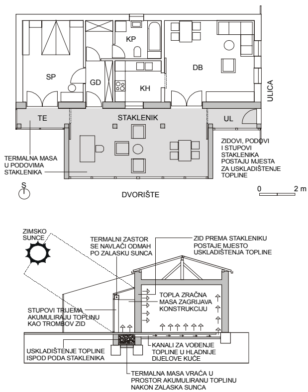
Slika 7. Tlocrt, presjek i izometrija solarne kuće
