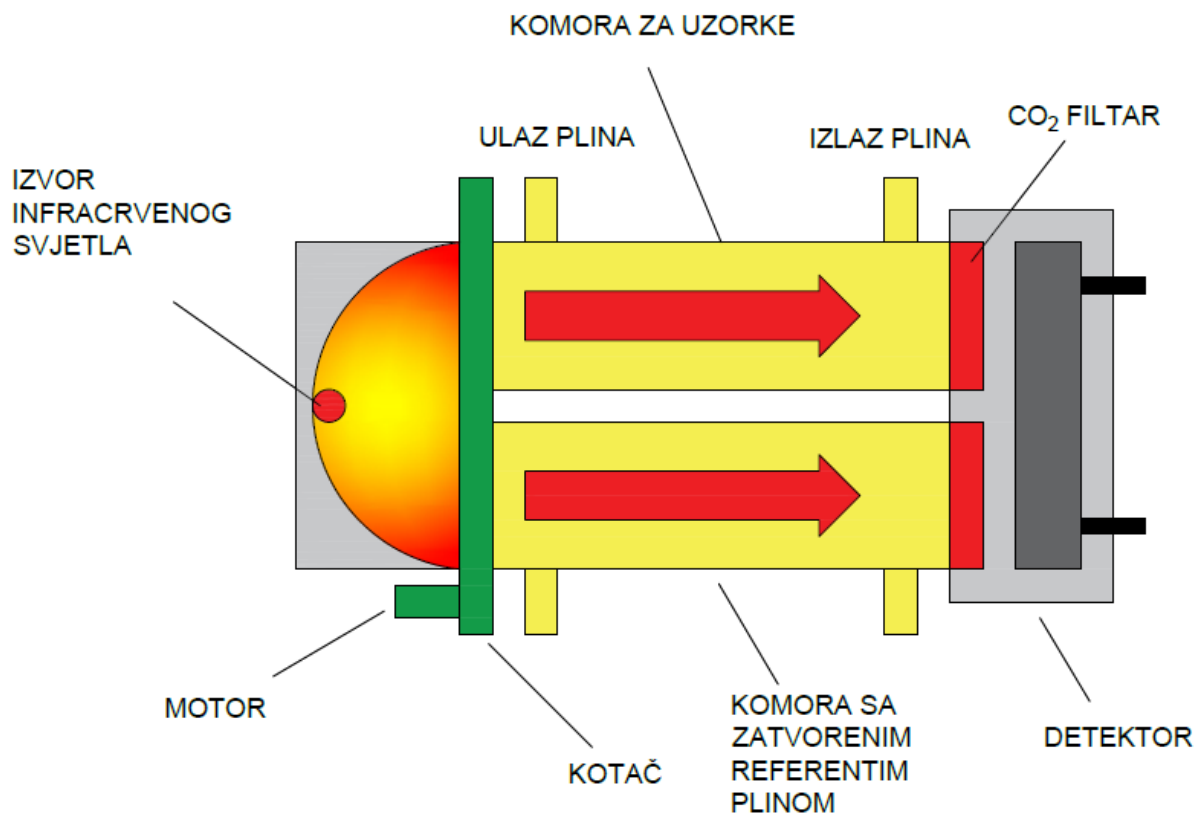
Sl. 2.29. – Princip rada infracrvenog senzora plina [24]
