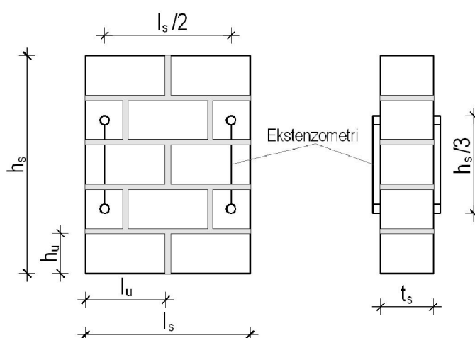
Slika 3.3–Uzorci zida za ispitivanje tlačne čvrstoće zida
