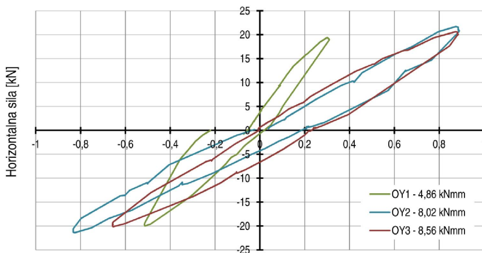
b) 2. ciklus opterećivanja
