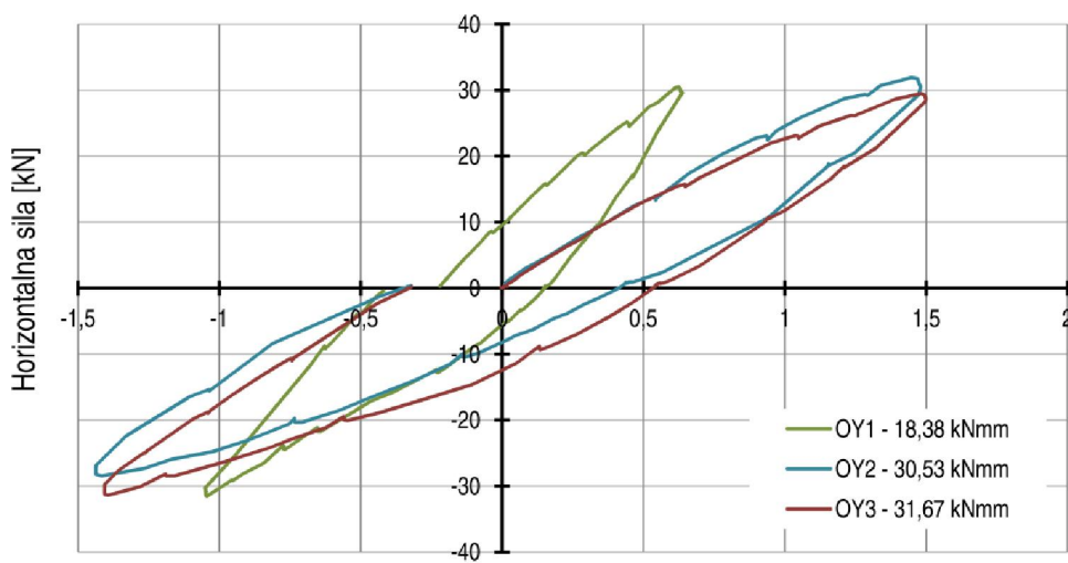
c) 3. ciklus opterećivanja
