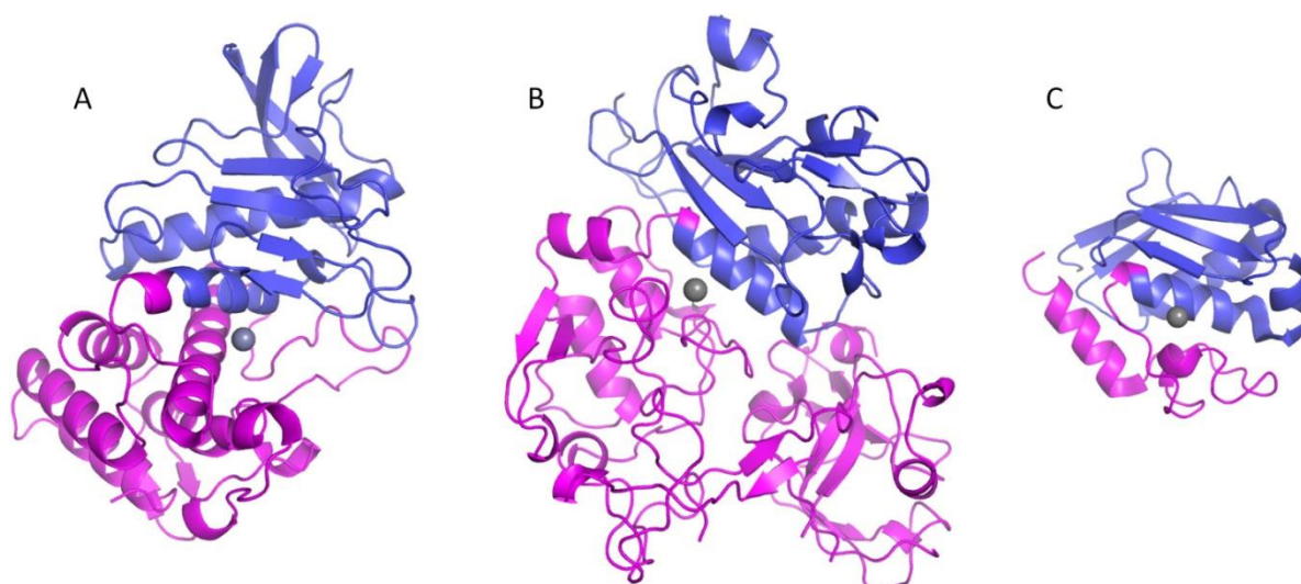
Slika 2.4. Primjeri raznolikosti C-terminalnih strukturnih domena iz klana peptidaza MA. Termolizin ( A ; PDB kod: 1TLX) i leishmanolizin ( B ; PDB kod: 1LML) su primjeri peptidaza s kompleksnim sekundarnim strukturama u C-terminalnoj strukturnoj domeni, dok ista domena u snapalizinu ( C ; PDB kod: 4HX3) sadrži samo jednu \alpha -zavojnicu i kratku petlju. Očuvana N-terminalna strukturna domena označena je plavo, a C-terminalna purpurnocrveno. Ion cinka prikazan je kao siva kuglica. Slika je pripravljena programom PyMol 52 .
