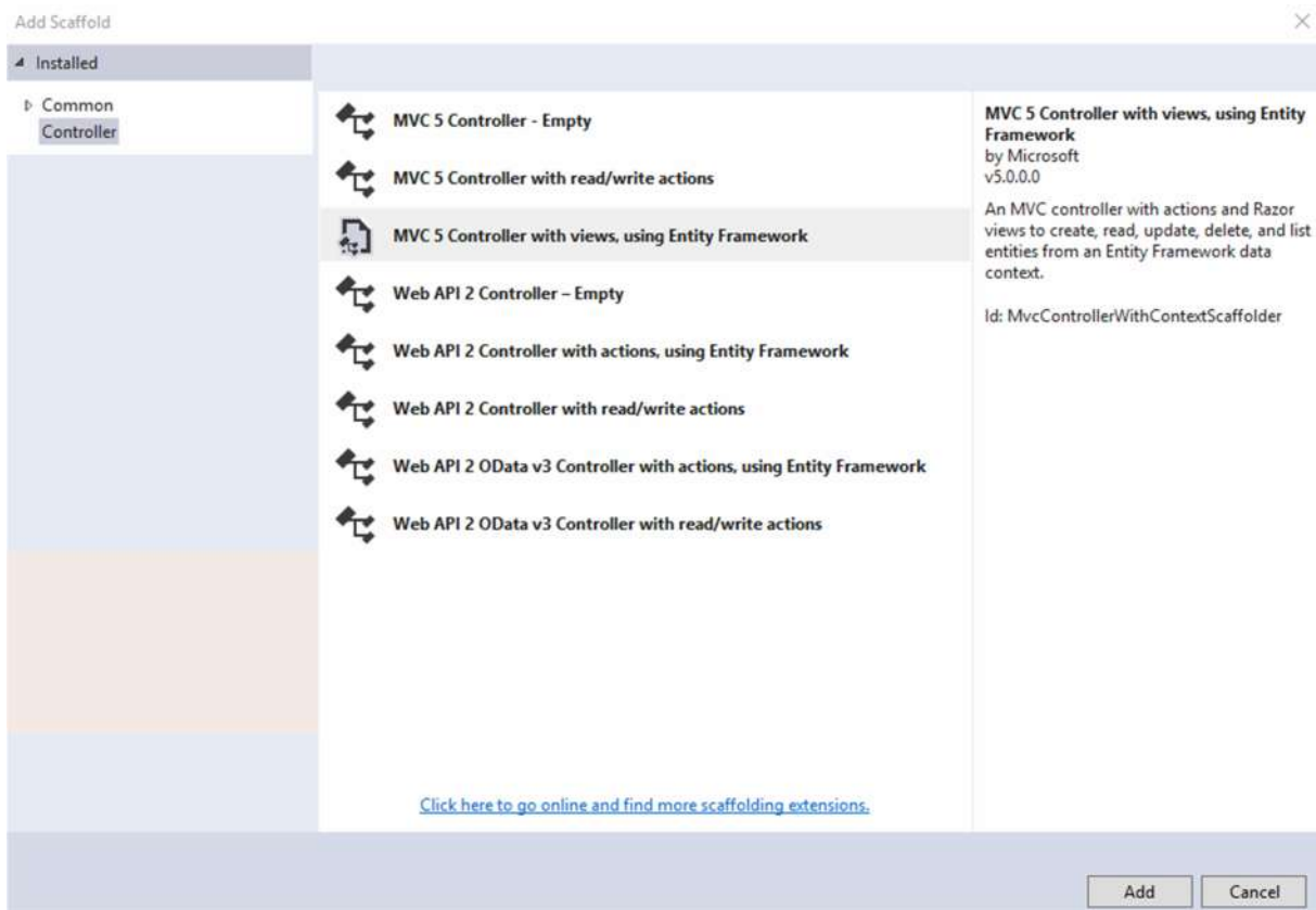
Slika 33. Odabir scaffold-a
