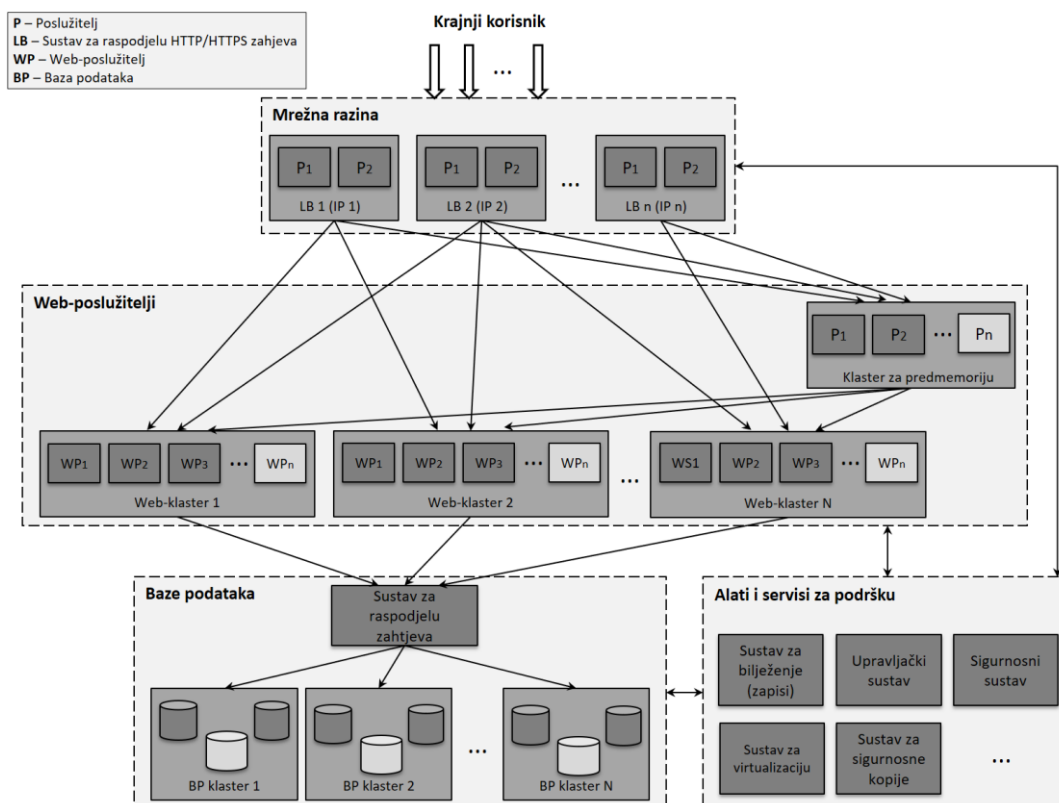
Slika 2.3. - Arhitektura Web-farme
