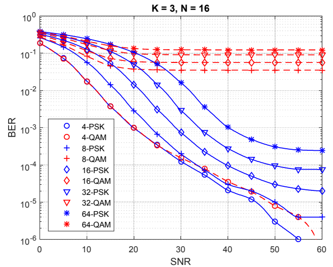
Slika 32: Vrijednosti BER-a pri određenim vrijednostima SNR-a uz K = 3 i N = 16
