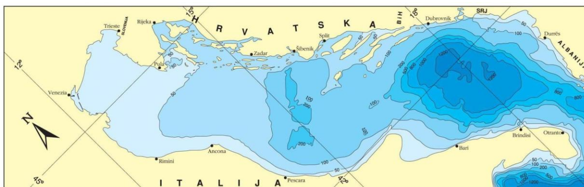
Slika 3.1. Batimetrijska karta Jadranskog mora.
