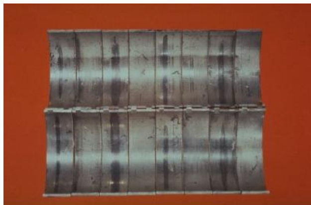
Slika 27. Adhezijsko trošenje zbog niske dobave ulja [6]
