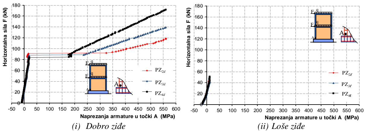
Slika 5.63. Utjecaj promjera vertikalnih šipki vertikalnih serklaža na naprezanje armature u točki A vertikalnog serklaža pri dnu zidanih zidova bez otvora
