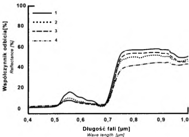
Ryc. 2. Zestawienie krzywych odpowiedzi spektralnej różnych roślin: 1 – podsadki wilczomlecza lancetowatego ( Euphorbia esula ), 2 – liście wilczomlecza, 3 – liście szczawiu kędzierzawego ( Rumex crispus ), 4 – mieszanka gatunkowa traw (za Parker Williams, Hunt 2004; zmienione).
