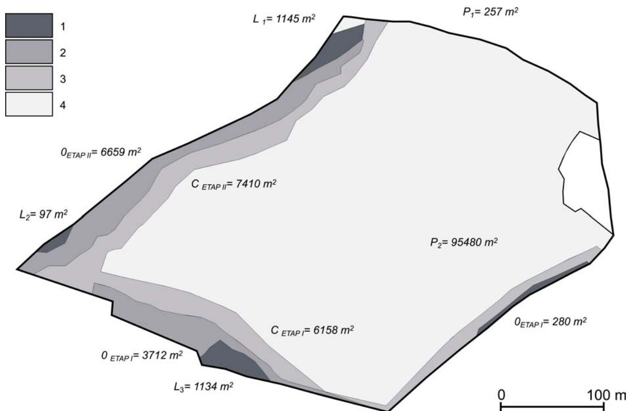
Rys. 1. Projekt rekultywacji dla OG „Obłaziec 1” (wg: Mapa sytuacyjno-wysokościowa, 1: 2000, Projekt rekultywacji, KSS Wisła S.A.):
