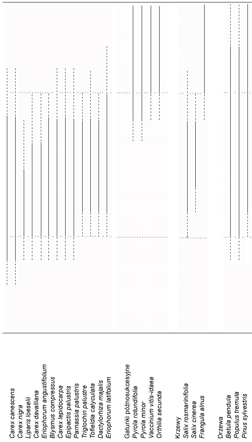
Rys. 2. Zmiany gatunków i następstwo zbiorowisk roślinnych podczas sukcesji w piaskowni Kuźnica Wąreżyńska (wg Rahmonov, Szymczyk, 2010)
