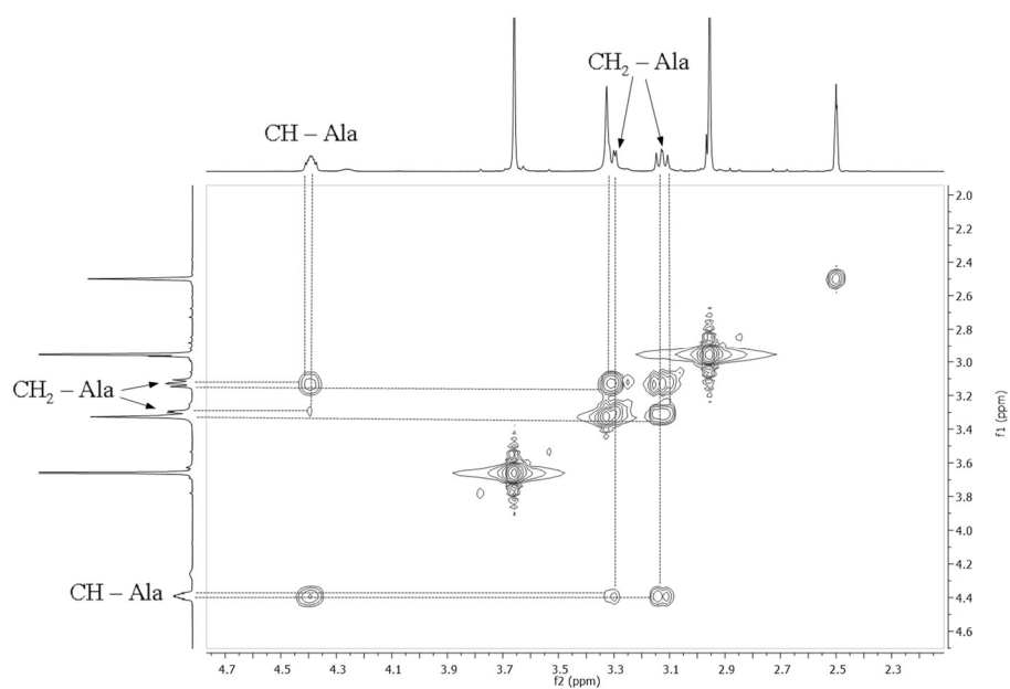
Slika 32. Dio COSY spektra 22 ; sprezanje CH 2 – Ala i CH – Ala te sprege CH 2 – Ala protona.
