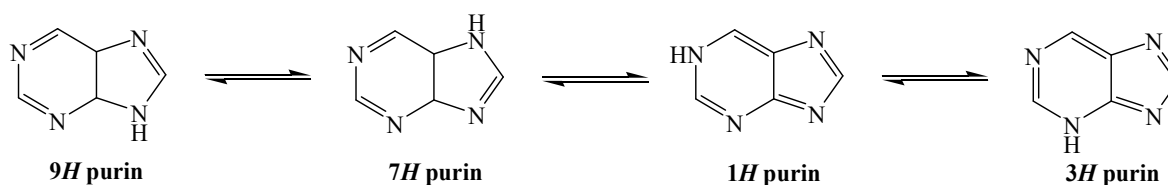
Shema 10. Tautomerne oblike purina.
