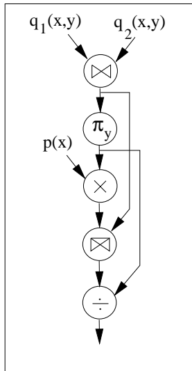
Ausdruck 1 (nach cnf)
