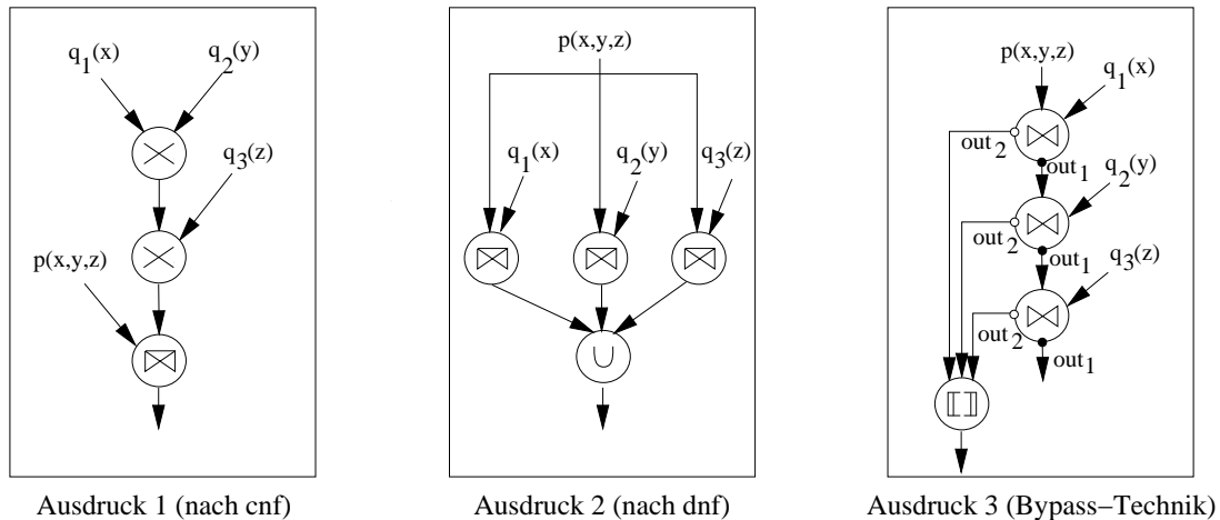
Abbildung 7: Alternative algebraische Ausdrücke Beispiel 2
