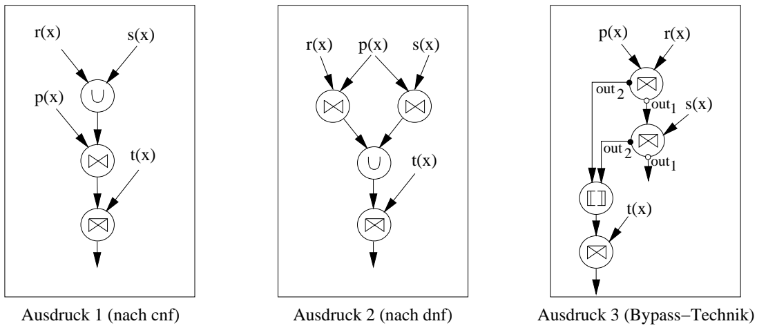
Abbildung 10: Alternative algebraische Ausdrücke Beispiel 1
