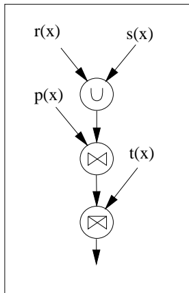
Ausdruck 1 (nach cnf)
