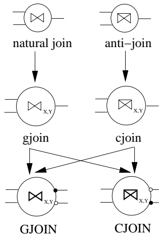
Abbildung 5: Verallgemeinerungshierarchie der Join-Operatoren
