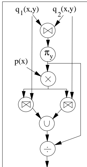
Ausdruck 2 (nach dnf)
