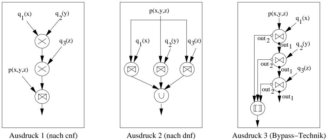
Abbildung 11: Alternative algebraische Ausdrücke Beispiel 2
