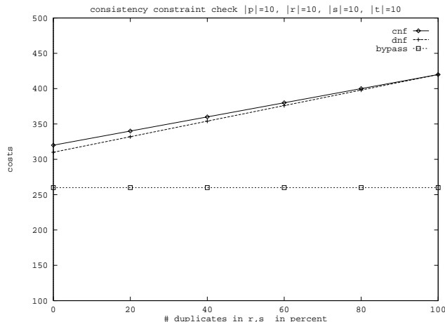
Abbildung 13: Kostenbetrachtung: Duplikate in Disjunktion
