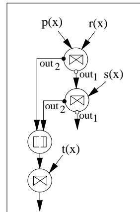
Ausdruck 3 (Bypass-Technik)
