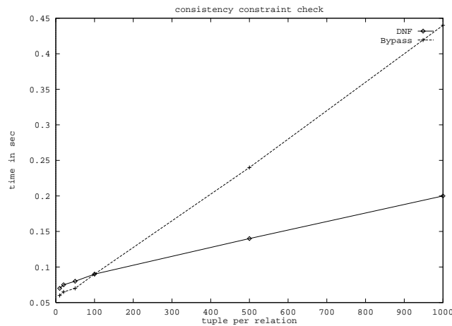
Abbildung 15: Benchmark Beispiel 2
