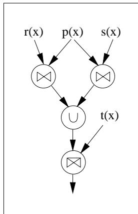
Ausdruck 2 (nach dnf)
