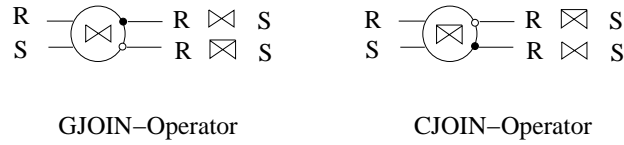
Abbildung 4: Verallgemeinerte Join-Operatoren mit 2 Ausgängen
