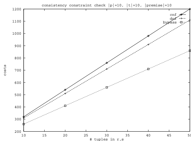
Abbildung 12: Kostenbetrachtung: Disjunktion in Prämisse
