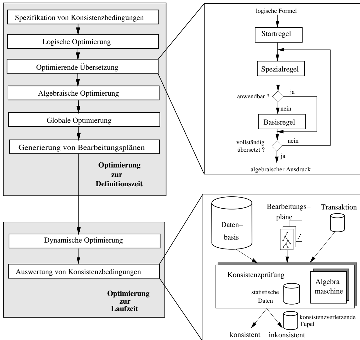
Abbildung 1: Gesamtsystem zur Konsistenzprüfung (Prinziplösung)
