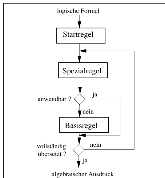
Abbildung 2: Übersetzungsprozeß
