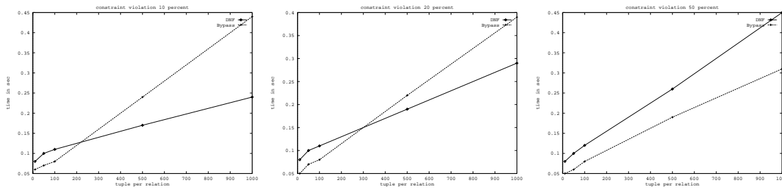
Abbildung 16: Benchmark Konsistenzverletzung
