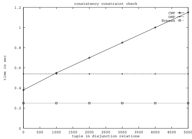
Abbildung 14: Benchmark Beispiel 1
