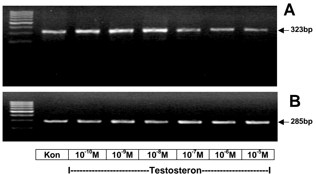
Abb. 4: Agarose-Gel mit den RT-PCR-Produkten der RBP-mRNA bei 323 bp (A) und der EF 1 \alpha -mRNA bei 285 bp (B) aus Hepatozyten von Xenopus laevis , die mit Konzentrationen von 10^{-10} M bis 10^{-5} M Testosteron behandelt sind. Die densitometrische Auswertung zeigt eine dosisabhängige Hemmung der RBP-mRNA-Synthese durch Testosteron auf ca. 40% der Kontrolle.
