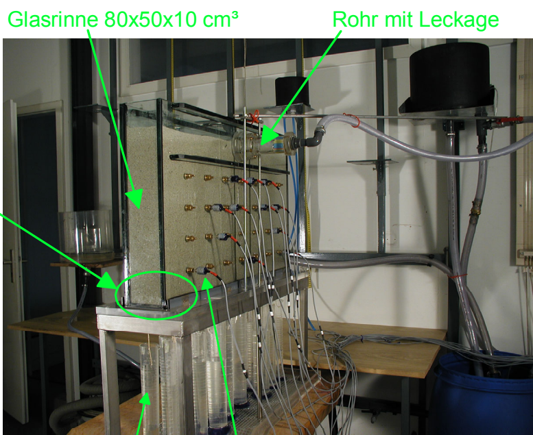
Messzylinder
