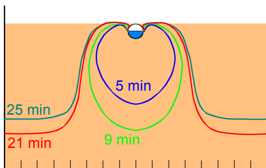
Abb. 2a: Zeitabhängiger Verlauf der Infiltrationsfront im Experiment
