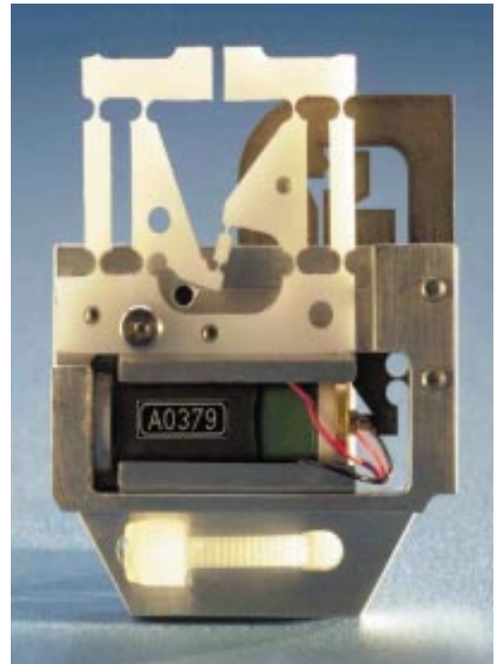
Abb. 6: Mikrogreifer mit monolithischer, wechselbarer Greifeinheit.
