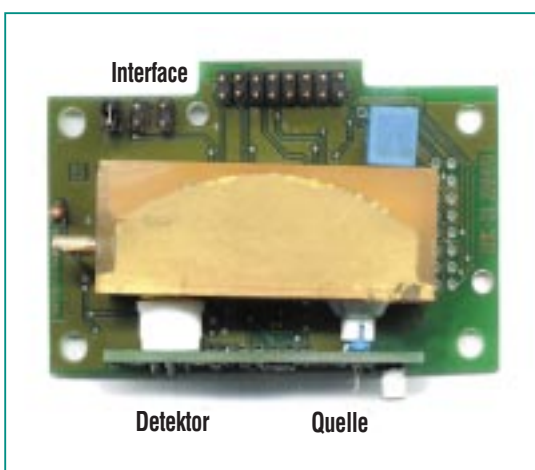
Abb. 2: Infrarot-Gassensor mit Controller-Interface.
