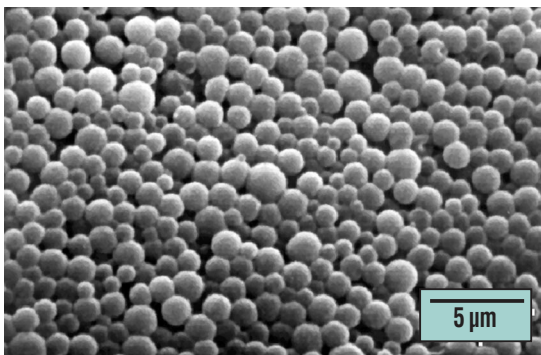
Abb. 3: Magnetische Polyvinylalkohol Mikropartikel der Firma chemagen Biopolymer-Technologie AG.
