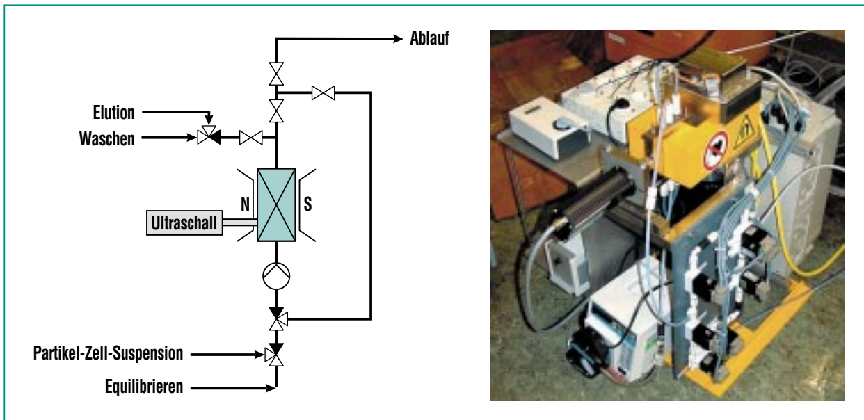
Abb. 5: Prototyp eines auf Magnettechnologie basierenden Aufreinigungssystems für Bioprodukte.
