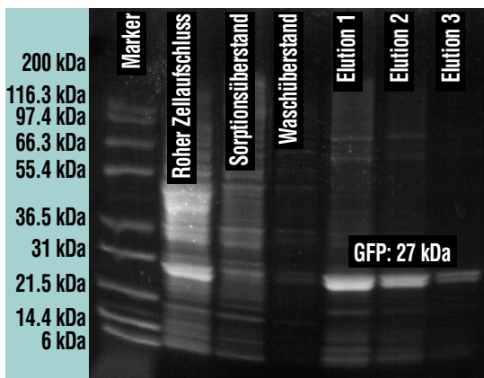
Abb. 6: Elektrophoresegel der Fraktionen eines Aufreinigungsversuchs: unterschiedliche Proteine werden nach ihrem Molekulargewicht (in kiloDalton notiert) aufgetrennt. Bahn 1: Standardisiertes Gemisch aus bekannten Proteinen zur Normierung, Bahn 2: Ausgangsmedium mit dem Zielprotein „Green Fluorescence Protein“ (GFP), Bahn 3: Überstand im Rührgefäß nach Zugabe der Sorbenspartikel, Bahn 4: Waschlösung nach Abtrennung der Sorbenspartikel im Separator, Bahn 5-7: Die Lösungen der drei Elutionsschritte sind weitgehend von Fremdproteinen befreit (vergleiche Bahn 2) und feststofffrei.
