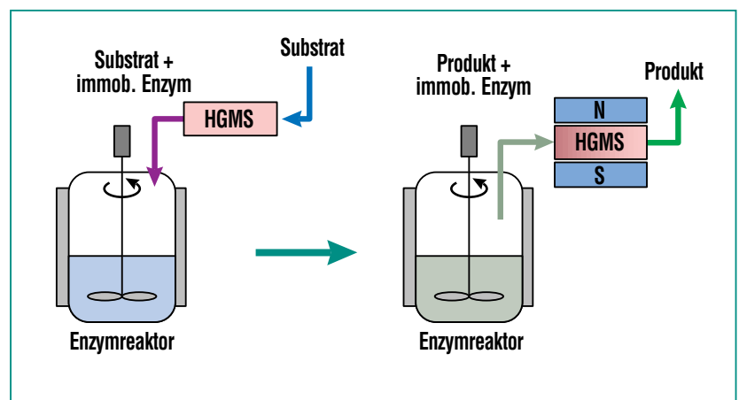
Abb. 4: Prinzip der Biokatalyse mit auf magnetischen Mikropartikeln immobilisierten Enzymen und Magnetseparatoren (HGMS).
