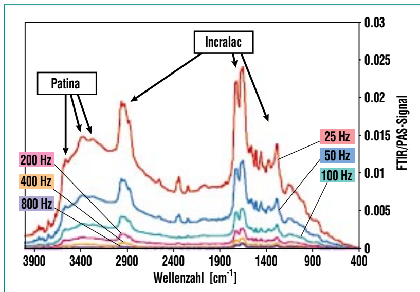
Abb. 3: FTIR/PAS-Tiefenprofil einer mit Incralac überzogenen Patina, wobei die mit verschiedenen Frequenzen aufgenommenen Spektren jeweils aus einer anderen Tiefe der Schicht stammen. In den Spektren kann deutlich zwischen den verschiedenen O-H-Absorptionsbanden der Patina (3588 bzw. 3580, 3402 und 3278 \text{cm}^{-1} ) und den C-H (2988 \text{cm}^{-1} ), C=O (1744 \text{cm}^{-1} ) und C-O-C (1242 und 1186 \text{cm}^{-1} ) Banden der aufgetragenen Incralac-Schutzschicht unterschieden werden.
