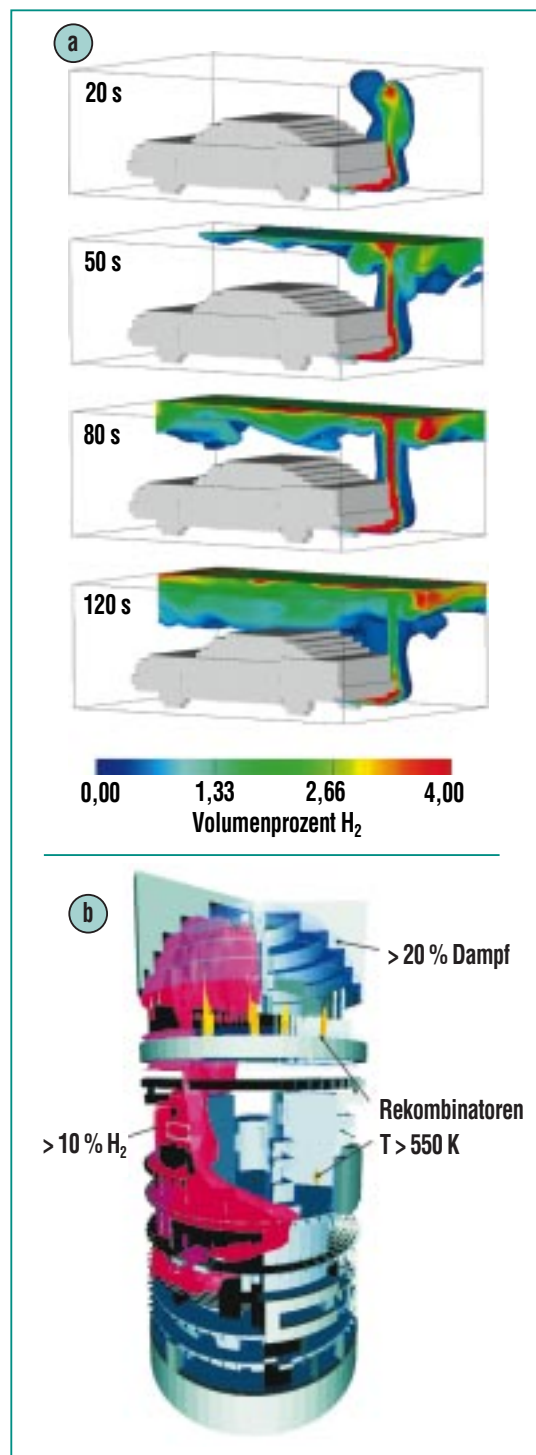
Abb.1: Simulation von Wasserstoff-Verteilungsprozessen mit dem 3D-Programm GASFLOW: a) H 2 -Fahrzeug in einer Garage; b) H 2 -Wolke in einem Reaktorsicherheitsbehälter.
