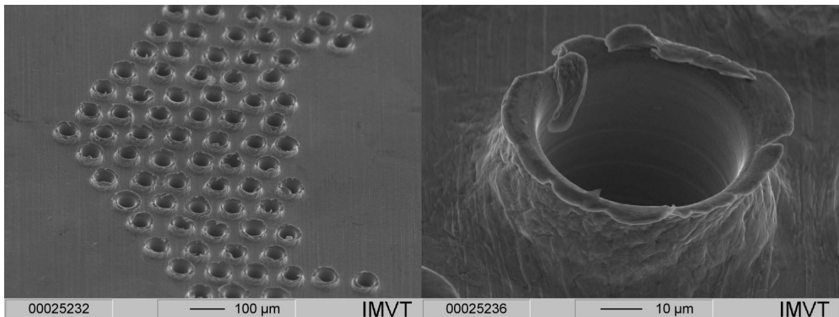
Abb. 12: Strukturelemente auf der Unterseite der Bedampfungsmaske mit massiven Graten durch plastische Verformung des Messings während des Mikrobohrens
