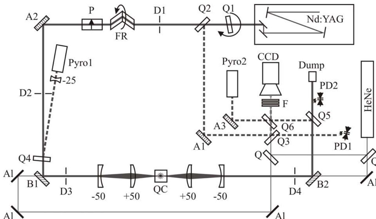
Abb. 3.5: Experimenteller Aufbau der LIBD-Instrumentierung.
