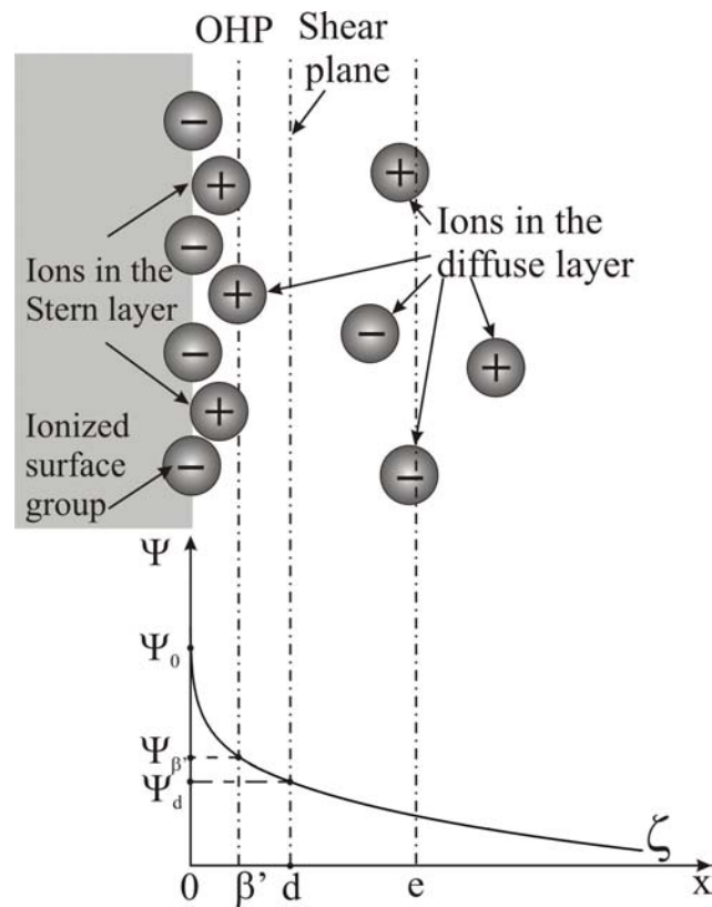
Abb. 2.1: Schematische Darstellung der Struktur der elektrischen Doppelschicht für den einfachen Fall eines Metalloxids im Grundelektrolyt. Die Oberflächenladung wird von ionisierten Oberflächen-Gruppen und/oder fest in der Stern-Schicht adsorbierten Ionen gebildet. Die dem Partikel zugewandte Ebene des diffusen Teils der elektrischen Doppelschicht wird äußere Helmholtz-Ebene (OHP) genannt. Die Scherfläche x = \beta' trennt die hydrodynamisch unbewegliche Flüssigkeit, die sich zusammen mit der Oberfläche bewegt x < \beta' von der beweglichen Flüssigkeit x > \beta' die sich bezüglich der Oberfläche mit endlicher Geschwindigkeit bewegt.
