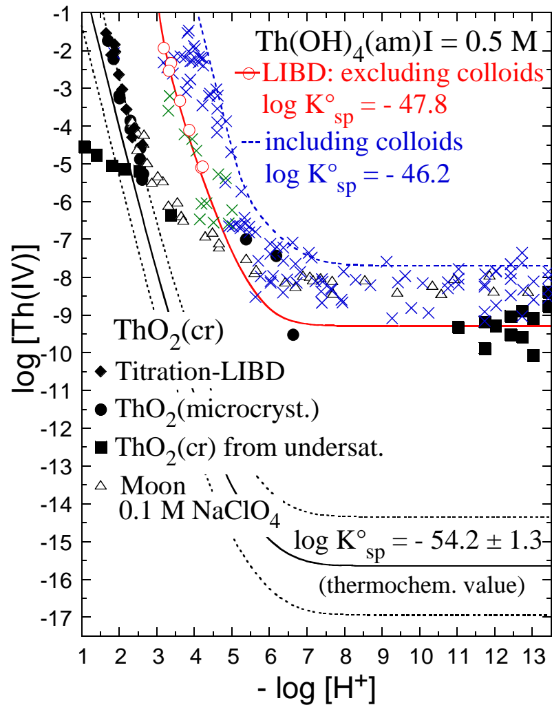
Abb. 5.1: Experimentelle und berechnete Löslichkeit von \text{ThO}_2(\text{cr}) und \text{Th(OH)}_4(\text{am}) . Die Löslichkeitsdaten für \text{ThO}_2(\text{cr}) wurden bei I = 0.5 \text{ M} ( \bullet ) und ( \blacksquare ) aus der Untersättigung [Nec 03], ( \blacklozenge ) durch coulometrische Titration / LIBD [Bun 00], bzw. bei I = 0.1 \text{ M} ( \triangle ) [Moo 89] bestimmt. Für die amorphen Festphasen \text{Th(OH)}_4(\text{am}) , die blaue Symbole ( \times ) stammen aus Löslichkeitsuntersuchungen bei I = 0.5 - 0.6 \text{ M} [Fel 91, Moo 89, Nab 64, Rya 87]. Eine gute Übereinstimmung ist zwischen den durch coulometrische Titration / LIBD [Nec 02] (die roten Punkten ( \circ )) und den von [Öst 94] (die grüne Symbole ( \times )) erhaltenen Löslichkeitsdaten bei I = 0.5 \text{ M} zu erkennen.
