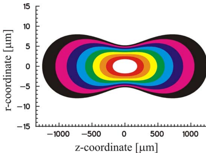
Abb. 3.3: Isolinien (Bereich von gleichem Photonenfluss, d.h. gleiche Flächenleistungsdichten) eines Laserpulses mit TEM_{00} -Profil im Fokusbereich.
