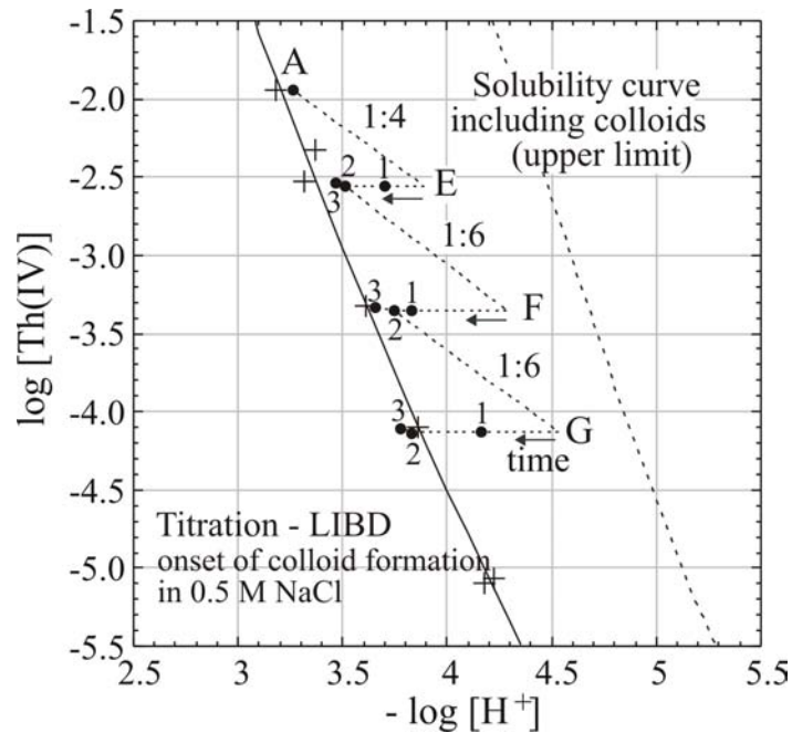
Abb. 5.7: \text{Th(IV)} - und \text{H}^+ -Konzentrationen in den kolloidalen \text{Th(IV)} -Suspensionen A – G (im Übersättigungsbereich).
