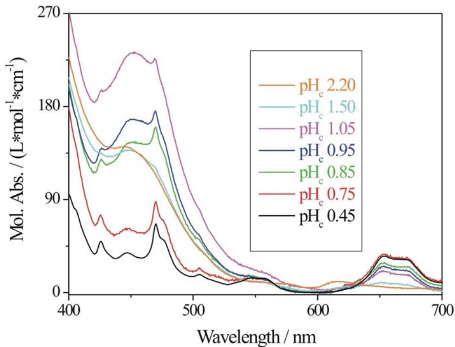
Abb. 6.22: Absorptionsspektren der durch Titration mit 1 M NaOH erhaltenen Pu-Lösungen mit Konzentrationen [Pu(IV)]_{tot} = 1.65 \cdot 10^{-4} - 3.18 \cdot 10^{-4} M und pH_c = 0.75 - 2.20 im Experiment A (s. Tabelle 8.4 des Anhangs).
