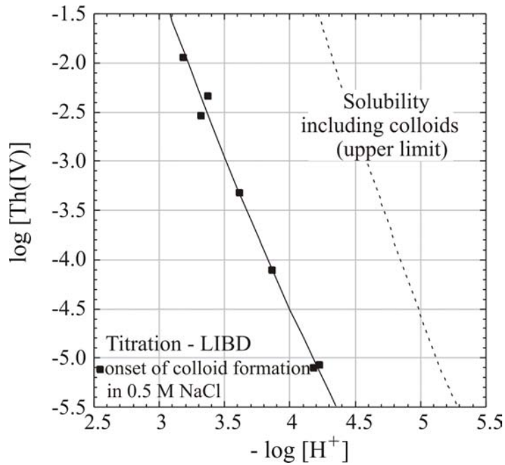
Abb. 5.2: Löslichkeit von \text{Th}(\text{OH})_4(\text{am}) bei I = 0.5 \text{ M} und 25^\circ\text{C} ; die durch coulometrische Titration / LIBD bestimmten experimentellen Daten (■) [Nec 02] entsprechen der unteren Löslichkeitskurve (ohne Beiträge von Kolloiden). Die gestrichelte Linie entspricht der Obergrenze von Löslichkeitsdaten (mit Beiträgen von Kolloiden). Die durchgezogene Kurve ist mit \log K_{\text{sp}}^\circ = -47.8 berechnet, die gestrichelte Linie mit \log K_{\text{sp}}^\circ = -46.2 sowie den Hydrolysekonstanten aus [Nec 01, Nec 02].
