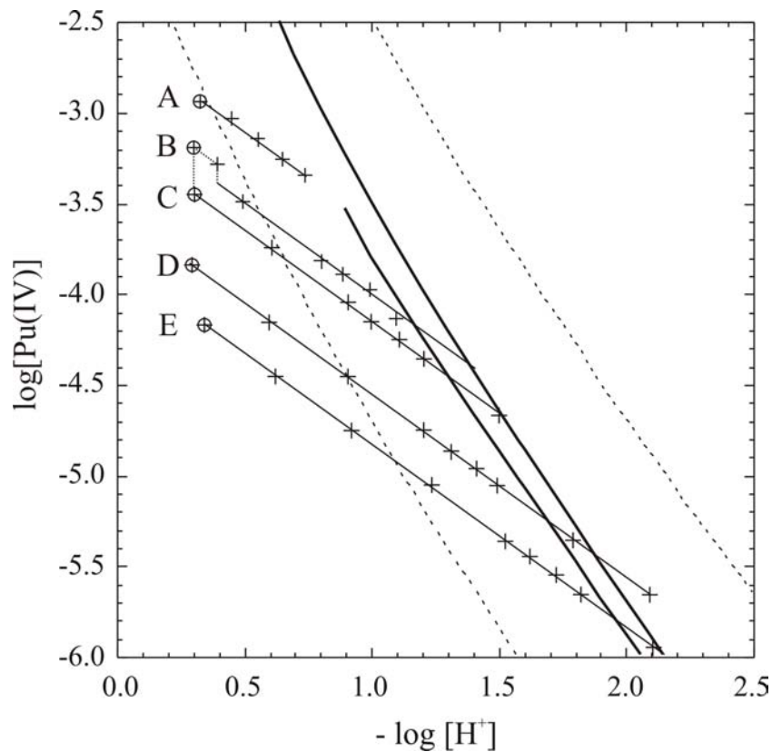
Abb. 6.5: Pu- und H^+ -Konzentrationen in den durch die Verdünnung-Titrationsexperimente A - E erhaltenen Pu-Lösungen.
