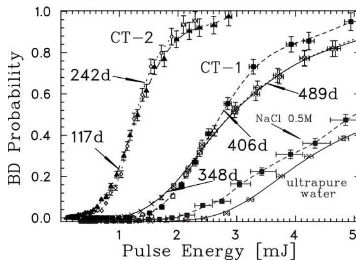
Abb. 5.14: LIBD-Untersuchungen der gealterten Th(IV)-Suspensionen CT-1 (niedrigste Konzentration [Th(IV)]_{coll} ) und CT-2 (höchste Konzentration [Th(IV)]_{coll} ) nach unterschiedlichen Zeiten.
