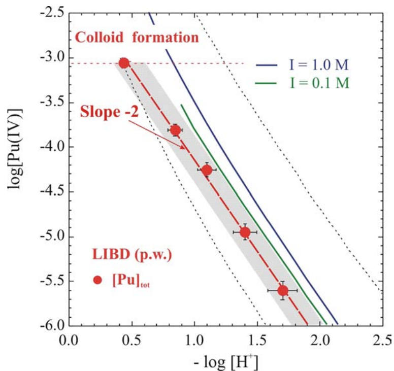
Abb. 6.17: Die durch Verdünnungstitrations mit 0.5 M NaCl und LIBD erhaltene Löslichkeitsdaten für Pu(OH) 4 (am) oder PuO 2 ·xH 2 O(am). Die durchgezogene Linien entsprechen den in [Nec 01] berechneten Löslichkeitskurven. Die gestrichelte Linien entsprechen dem Unsicherheitsbereich der Literatur-Löslichkeitsdaten. Der graue Keil zeigt den mit LIBD erhaltenen Unsicherheitsbereich.
