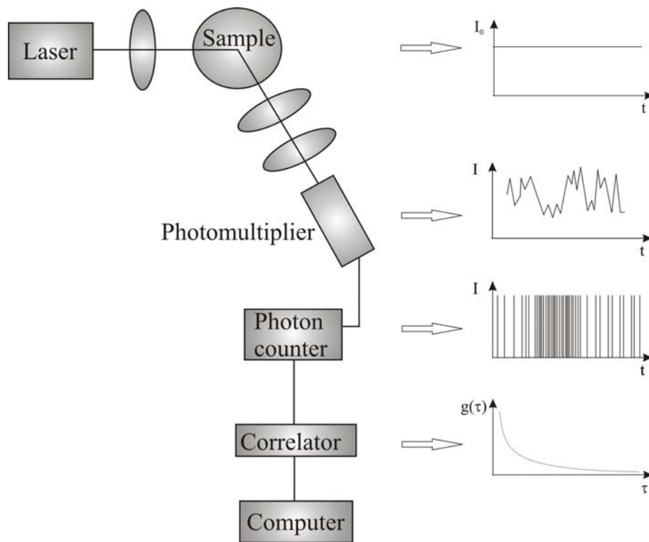
Abb. 2.4: Schematischer Aufbau der Photonenkorrelationspektroskopie-Instrumentierung bestehend aus: Laser (Lichtquelle), Messzelle und Photomultiplier. Der Photomultiplier gibt die Signale einer Messelektronik (Korrelator und PC) weiter. Mit dem Korrelator werden die zeitlichen Schwankungen der Streulichtintensität erfasst und vom PC ausgewertet.
