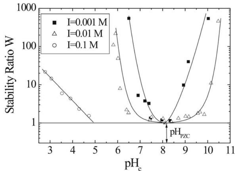
Abb. 4.2: Stabilitätsverhältnis von 140 nm ZrO_2 -Kolloiden bei verschiedenen Ionenstärken als Funktion des pH_c -Wertes.
