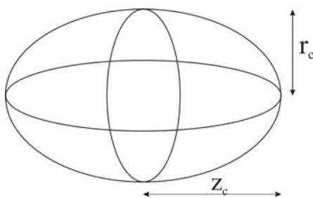
Abb. 3.2: Annäherung des Laserfokus durch einen Rotationsellipsoiden.
