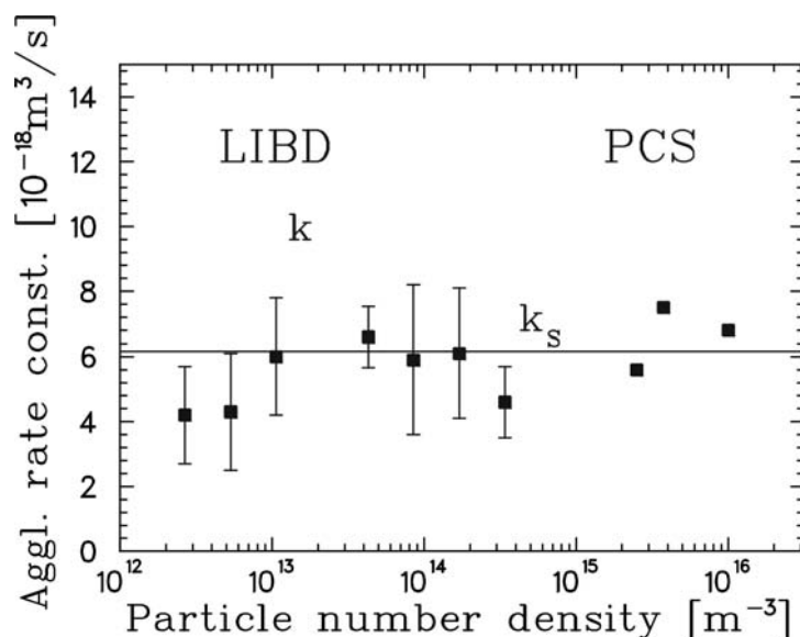
Abb. 4.7: Die mit der LIBD und PCS bestimmten Agglomerationsratenkonstanten als Funktion der Partikelanzahldichte. Vergleich mit der Smoluchowsky-Konstante.
