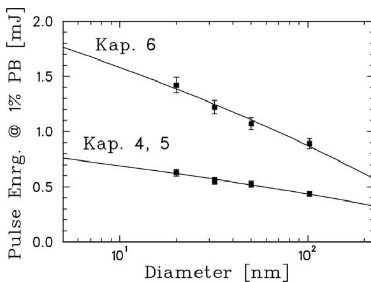
Abb. 8.3: Die mit Polystyrol-Partikeln erhaltene Kalibrationskurve der LIBD-Instrumentierung, welche für die in Kapitel 6 beschriebene Untersuchungen zur Hydrolyse und Kolloidbildung von Pu(IV) verwendet wurde. Vergleich zur Kalibrationskurve der LIBD-Instrumentierung für die in Kapitel 4 und 5 beschriebene Untersuchungen (ZrO 2 , bzw. Th(OH) 4(am) -Kolloide).
