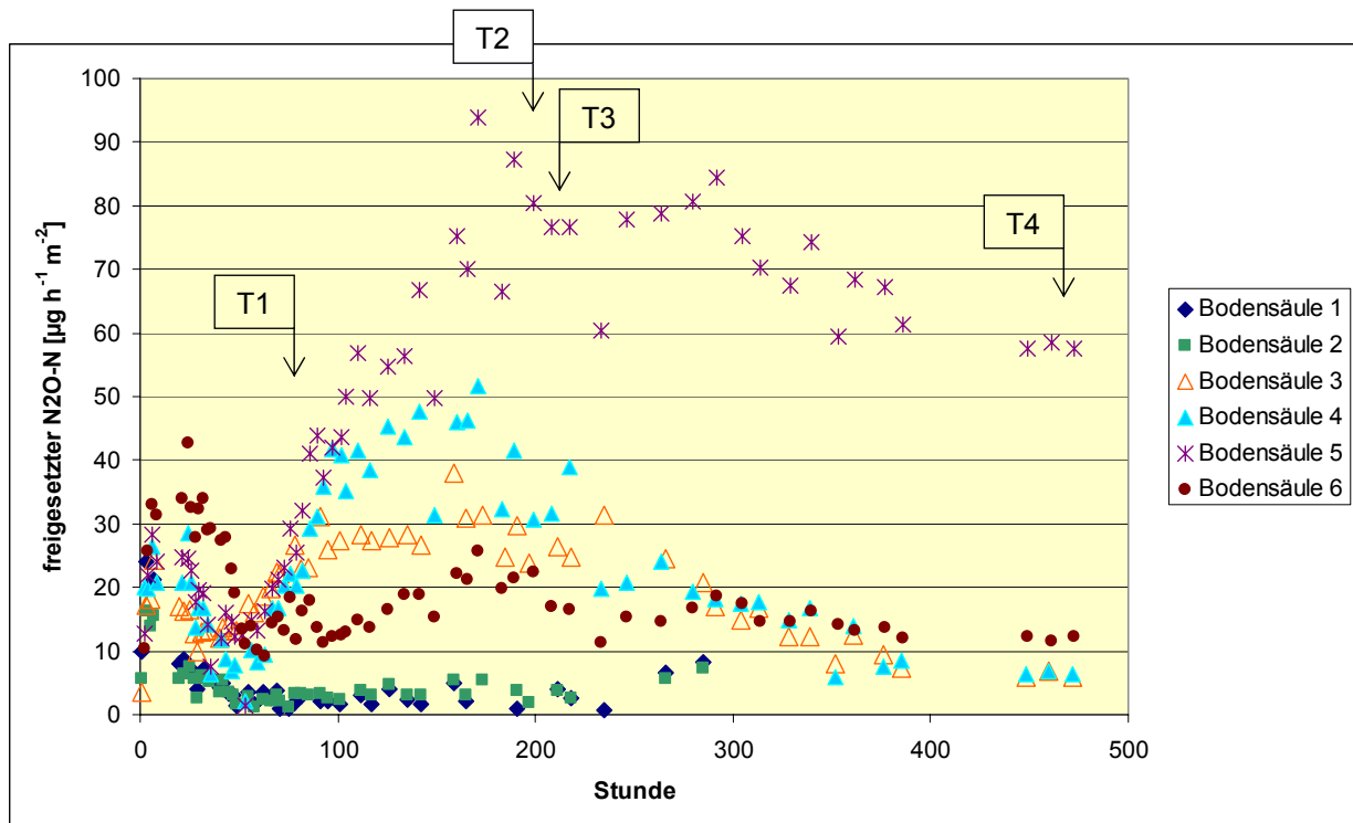
Abbildung 4-1: N 2 O-Emission [µg N m -2 h -1 ] aus Bodensäulen während und nach dem Auftauen. Dargestellt sind die Werte der einzelnen Bodensäulen aus der zweiten Versuchsreihe. Die Berechnung erfolgte nach der im Text beschriebenen Formel. Die Zeitpunkte der Bodenprobenentnahmen (T1 bis T4) sind eingezeichnet.
