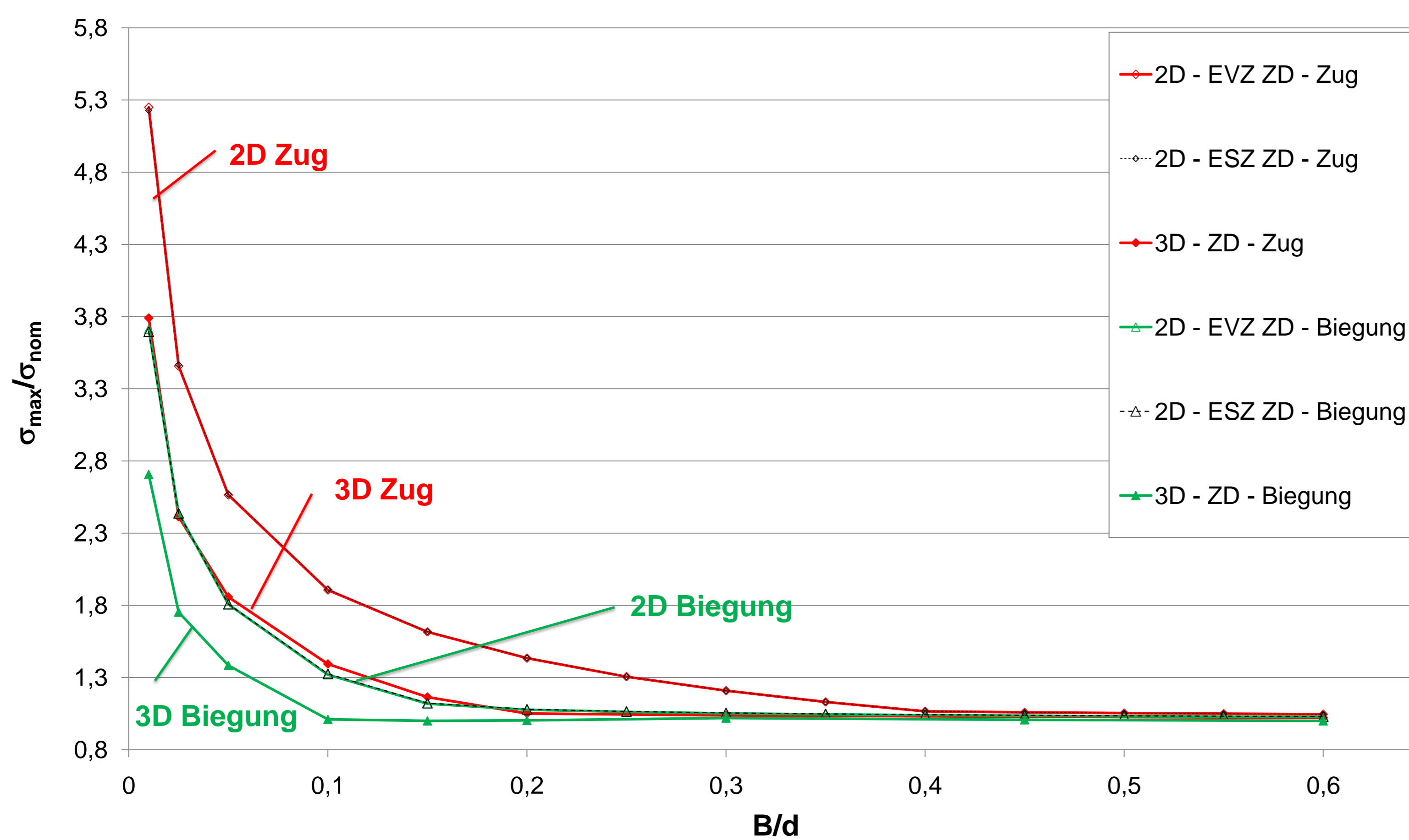
D=300, d/D= 1/3, Zug maximale v. Mises Vergleichsspannung
