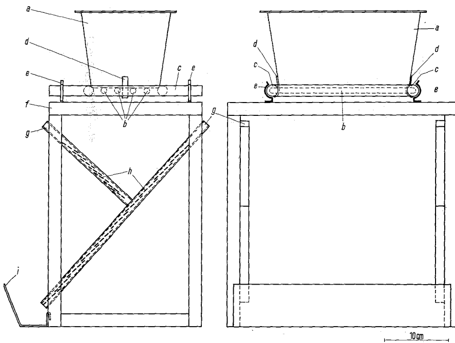
Abb. 2. Seitenriß und Aufriß des Stoffwechsellkäfigs. Einzelheiten s. Text.
