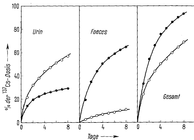
Abb. 1. Kumulative Ausscheidung von intraperitoneal injiziertem ^{137}\text{Cs} bei Kontrollratten und bei Verfütterung von 1% BB. Mittelwerte von je 6 Weibchen mit einem mittleren Körpergewicht von 190 g.
