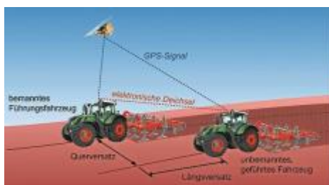
Konzept der elektronischen Deichsel
