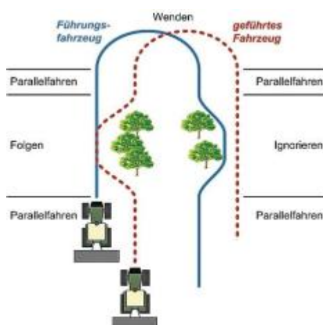
Fahrmodi zur Bedienung der elektronischen Deichsel
