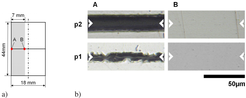
Figure 6.15: Variation des Diffusionsschweißdrucks. a) Skizze der betrachteten Positionen in der Schweißnaht. b) Lichtmikroskopische Aufnahmen der diffusionsgeschweißten Proben. Die verwendeten Prozessparameter können Tabelle 6.4 entnommen werden.
