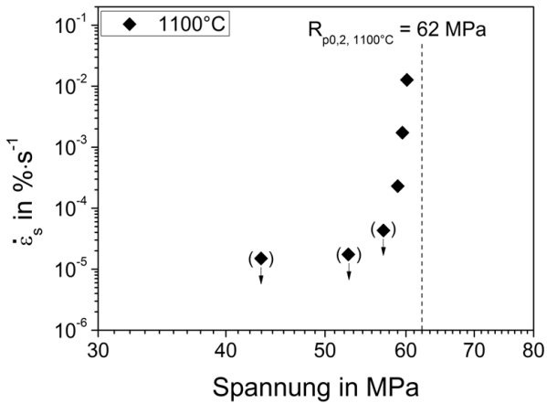
Abbildung 4.15: Zugkriechversuche bei 1100^\circ C . Die stationäre Kriechrate der eingeklammerten Versuchspunkte liegt unterhalb der eingezeichneten.
