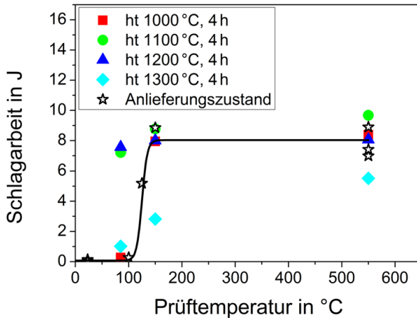
Abbildung 4.11: Kerbschlagzähigkeiten des Ausgangsmaterials sowie ausgelagerter Proben. Oberhalb einer Wärmebehandlungstemperatur von 1200 °C erfolgt ein Zähigkeitsverlust.
