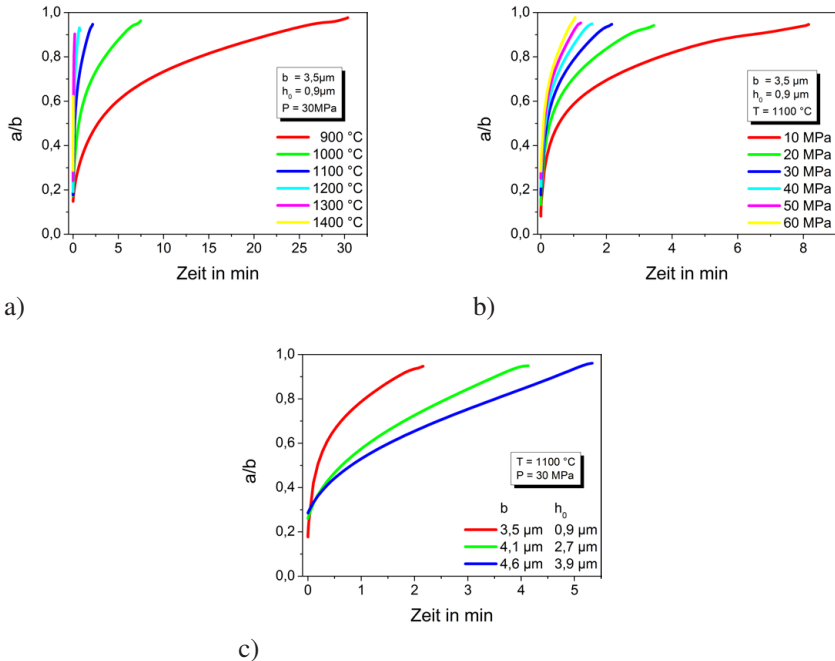
Abbildung 5.10: Modellierung der Hohraumschließung. a) Eine Temperaturerhöhung beschleunigt den Diffusionsschweißprozess ebenso wie b) eine Druckerhöhung oder c) eine Verminderung der Oberflächenrauheit.
