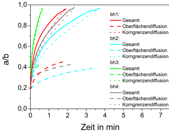
Figure 6.10: Simulation der Hohlraumschließung mit den Parametersätzen aus Tabelle 6.3. Eine gröbere Oberflächenrauheit führt zu einer längeren erforderlichen Diffusionsschweißzeit.
