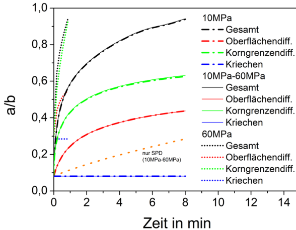
Abbildung 5.11: Die lineare Druckerhöhung während des Diffusionsschweißprozesses führt zu einer Beschleunigung des Fügevorgangs von 6s. Die verwendeten Simulationsparameter sind b = 3,5\ \mu\text{m} , h_0 = 0,9\ \mu\text{m} und T = 1100^\circ\text{C} .
