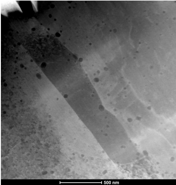
Figure 6.3: STEM Aufnahme der Diffusionsschweißnaht. Es können keine Partikelagglomerationen beobachtet werden und die Oxidpartikel sind homogen in den (Sub-)Körnern verteilt ohne sich an den Korngrenzen anzusammeln.
