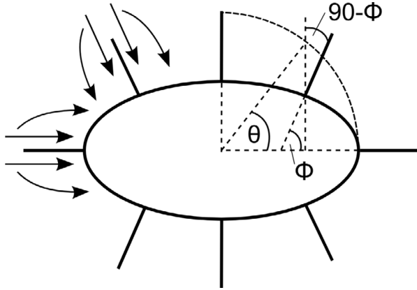
Abbildung 5.4: Schematische Darstellung der Wirkungsweise von Korngrenzen am elliptischen Hohlraum. Bei einer kleinen Korngröße, im Verhältnis zur Breite der Einheitszelle, kann entlang mehrerer Korngrenzen Materialtransport erfolgen; adaptiert nach [13]
