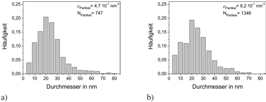
Abbildung 4.2: Partikelgrößenverteilungen von PM2000 im Anlieferungszustand. a) Mitte des Rundstabs und b) Randbereich des Rundstabs.
