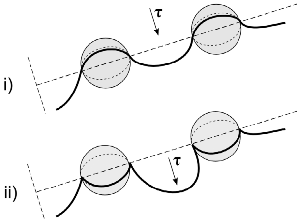
Abbildung 2.4: Schematische Darstellung des Kletterprozesses (i) und Interfacial Pinnings (ii). Der Kletterprozess beschreibt, wie eine Versetzung über einen Partikel klettert und nach dem Überklettern stark an der Partikel/Matrix Grenzfläche anhaftet; adaptiert nach [17].
