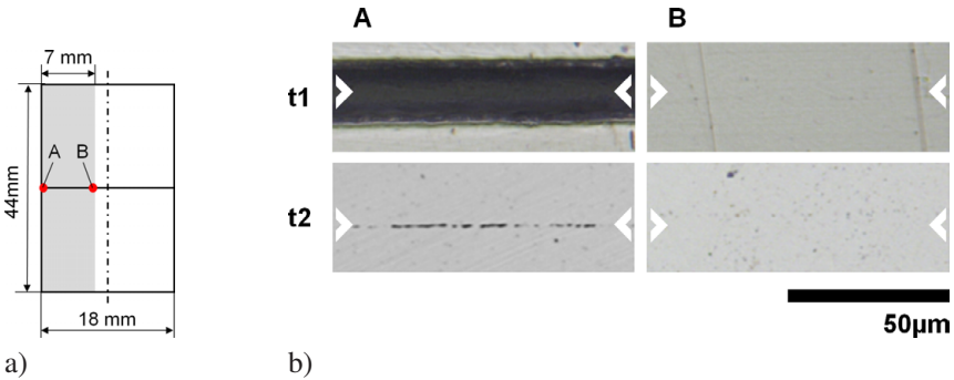
Figure 6.6: Variation der Diffusionsschweißzeit. a) Skizze der betrachteten Positionen in der Schweißnaht. b) Lichtmikroskopische Aufnahmen der diffusionsgeschweißten Proben. Die verwendeten Prozessparameter können Tabelle 6.1 entnommen werden.
