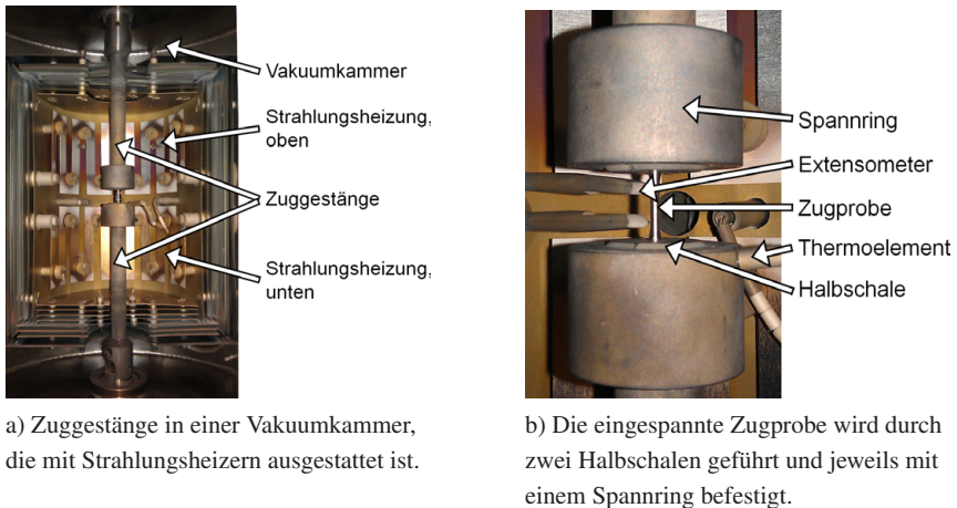
Figure 3.2: Fotografische Abbildung der Zugprüfanlage: a) Übersichtsaufnahme und b) Detailaufnahme der Probenspannvorrichtung und Dehnungsmessvorrichtung.
