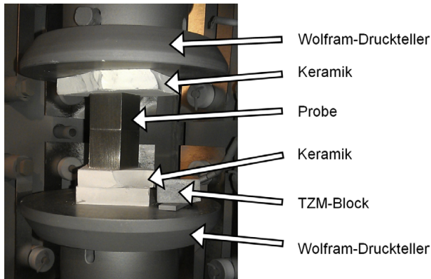
Figure 3.5: Fotografische Abbildung der Versuchsanordnung während einer Diffusionsschweißung.
