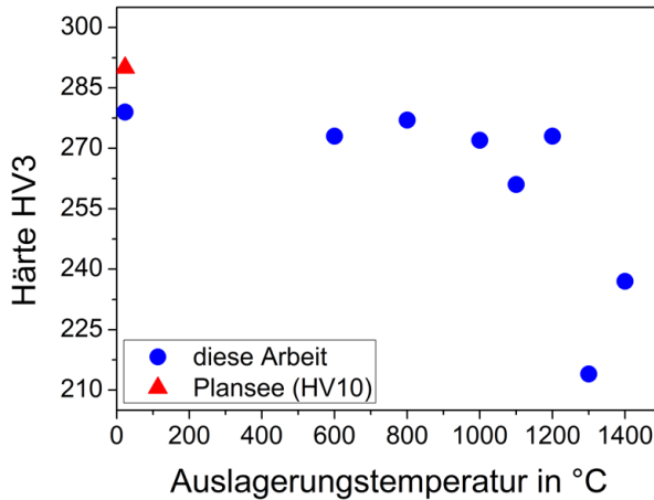
Abbildung 4.9: Einfluss der Auslagerungstemperatur auf die Vickershärte. Die ermittelte Härte im Anlieferungszustand ist vergleichbar mit den Herstellerangaben [61]. Oberhalb einer Auslagerungstemperatur von 1200°C verringert sich die Härte um 22%.
