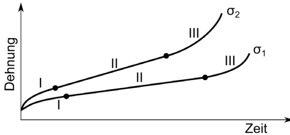
Abbildung 2.1: Dehnungsverhalten aufgetragen über die Zeit für zwei Spannungen, mit \sigma_2 > \sigma_1 bei konstanter Temperatur. Es bilden sich drei Kriechbereiche aus, das primäre (I), sekundäre (II) und tertiäre (III) Kriechen; adaptiert nach [35, 36].
