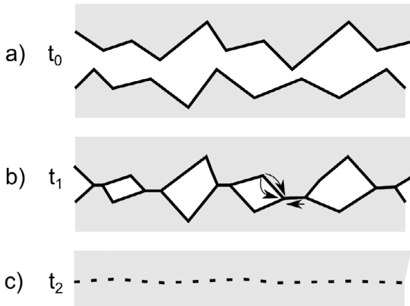
Abbildung 2.7: Prinzipskizze des zeitabhängigen Diffusionsschweißprozesses. a) Die Oberflächen vor der Ausübung einer Druckspannung. b) Die Druckspannung verformt die Rauheitsspitzen plastisch, Kriechprozesse können ebenfalls beteiligt sein. Die Diffusionspfade entlang der Hohlraumoberfläche und der Korngrenze sind eingezeichnet. Die Pfeilrichtung kennzeichnet die Richtung des Materialtransports. c) Erfolgreiche Diffusionsschweißverbindung.
