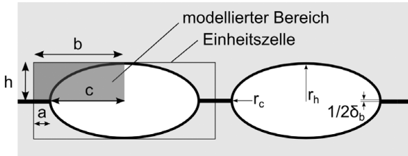
Abbildung 5.1: Die modellierte Fläche beträgt, aufgrund der zwei Symmetrieachsen, ein Viertel des elliptischen Hohlraums. Die Hälfte der Rauheitswellenlänge wird mit b beschrieben, die kurze Halbachse der Ellipse mit h und der bereits verbundene Bereich mit a . Rechts ist der Krümmungsradius der langen Halbachse r_c und der kurzen Halbachse r_h der Ellipse, wie auch die Korngränzschieblage \delta_b eingezeichnet; adaptiert nach [13].
