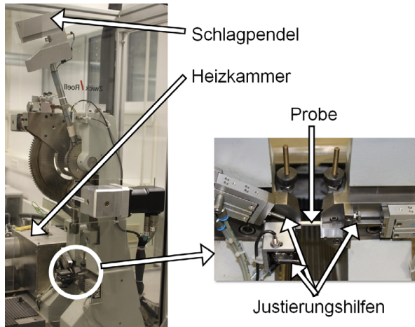
Figure 3.3: Fotografie der verwendeten Kerbschlagbiegeprüfanlage.
