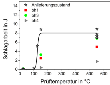
b) Kerbschlagbiegeversuche
