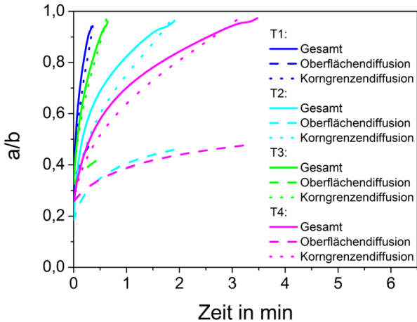
Figure 6.7: Variation der Diffusionsschweißtemperatur. Simulation der Hohlräume schließung mit den Parametersätzen aus Tabelle 6.2. Eine höhere Diffusionsschweißtemperatur führt zu einer schnelleren Schließung des Hohlraums.
