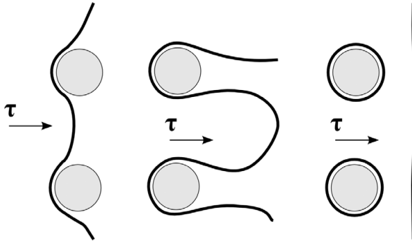
Abbildung 2.3: Schematische Darstellung des Orowan Mechanismus. Der Orowan Mechanismus beschreibt wie eine Versetzung von einem Partikel aufgehalten wird. Sie umschlingt den Partikel und bildet sich nach dem Partikel neu, es bleibt ein Orowan Ring zurück; adaptiert nach [35].
