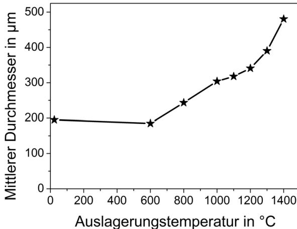
Abbildung 4.6: Kornwachstum nach Auslagerungen, in einem Temperaturbereich von 600°C bis 1400°C für jeweils 4h. Das verwendete PM2000 weist ein bimodales Korngefüge auf. Die größeren Körner liegen im Bereich einiger Millimeter und sind in diesem Diagramm nicht erfasst. Die kleineren Körner zeigen ein Wachstum von etwa 200µm auf 480µm.
