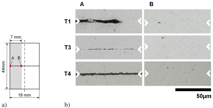
Figure 6.9: Variation der Diffusionsschweißtemperatur. a) Skizze der betrachteten Positionen in der Schweißnaht. b) Lichtmikroskopische Aufnahmen der diffusionsgeschweißten Proben. Die verwendeten Prozessparameter sind in Tabelle 6.2 aufgeführt.
