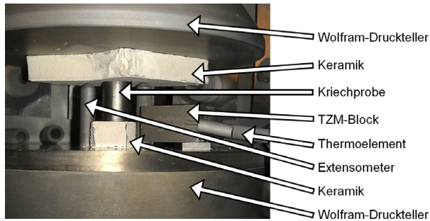
Figure 3.4: Fotografische Abbildung des Kriechversuchs.
