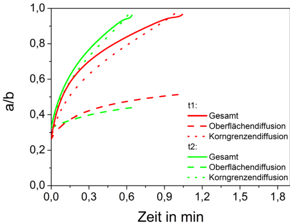
Figure 6.4: Simulation der Hohlräume für die Parametersätze aus Tabelle 6.1. Die leicht unterschiedlichen Oberflächenrauheiten führen zu einem unterschiedlichen Einfluss der spontanen plastischen Deformation.
