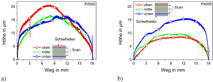
Figure 6.1: Oberflächenrauheitsprofil der zu verschweißenden Proben, es werden drei Messungen pro Probe durchgeführt. Die Breite und Höhe des modellierten Bereichs betragen a) b = 4,1 \mu\text{m} , h_0 = 1,3 \mu\text{m} , b) b = 3,2 \mu\text{m} und h_0 = 0,9 \mu\text{m} .
