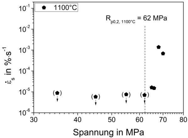
Abbildung 4.14: Druckkriechversuche bei 1100^\circ C . Die Spannungsabhängigkeit der Kriechrate beginnt knapp oberhalb der Dehngrenze bei 1100^\circ C . Die stationäre Kriechrate der eingeklammerten Versuchspunkte liegt unterhalb der eingezeichneten.
