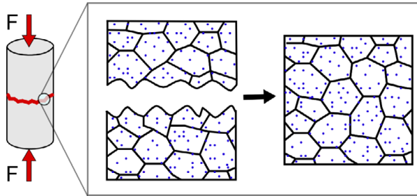
Abbildung 2.5: Schematische Darstellung des Diffusionsschweißprozesses. Bei erhöhter Temperatur werden die Füge­teile eine hinreichend lange Zeit aufeinander gepresst. Während dieser Zeit bildet sich, aufgrund von Verformungs- und Diffusionsprozessen, ein nahtloses Gefüge aus. Die blauen Punkte symbolisieren die Oxidpartikel.
