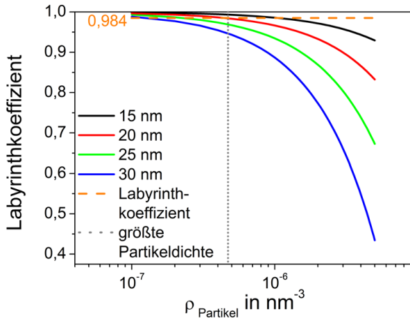
Abbildung 5.5: Bestimmung des Labyrinthkoeffizienten in Abhängigkeit der Partikeldichte und des mittleren Partikeldurchmessers.
