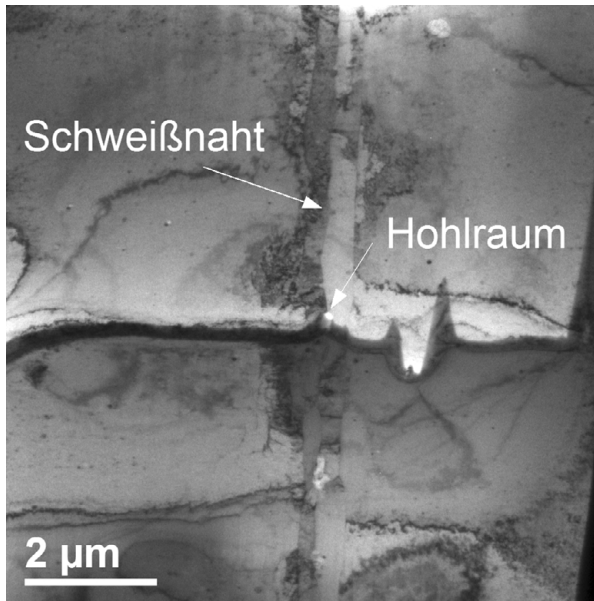
Figure 6.2: TEM Hellfeldaufnahme einer Diffusionsschweißnaht. Die Schweißnaht verläuft senkrecht und die waagerechte Linie trennt zwei unterschiedlich dicke Bereiche der TEM Lamelle, die sich aus der Probenpräparation ergeben.
