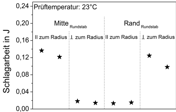
Abbildung 4.4: Kerbschlagbiegeversuche bei 23°C. Es wird Material vom Rand und aus der Mitte des Rundstabs untersucht. In beiden Bereichen wird zwischen Proben mit einem Kerb parallel bzw. senkrecht zum Rundstabsradius unterschieden und jeweils 2 Proben getestet. Der Einfluss der Orientierung des Kerbs ist größer als der Einfluss der Entnahmeposition. Bei Raumtemperatur weist PM2000 ein sprödes Verhalten auf.
