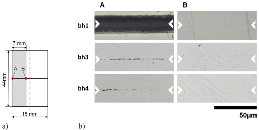
Figure 6.12: Variation der Oberflächenrauheitskennwerte. a) Skizze der betrachteten Positionen in der Schweißnaht. b) Lichtmikroskopische Aufnahmen der diffusionsschweißten Proben. Die verwendeten Prozessparameter können Tabelle 6.3 entnommen werden.
