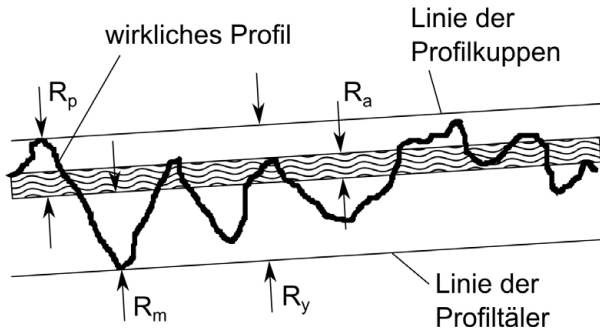
Abbildung 2.8: Schematische Darstellung der Oberflächenrauheit, das Rauheitsprofil ist fett eingezeichnet. R_p : maximale Profilkuppenhöhe, R_m : maximale Profiltiefe, R_y maximale Profilhöhe, R_a arithmetischer Mittenrauhwert; adaptiert nach [95].
