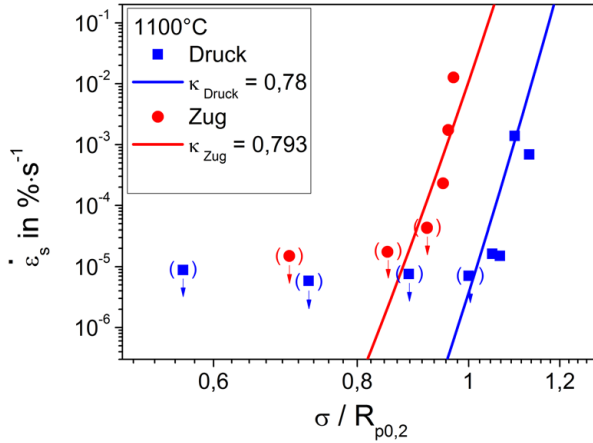
Abbildung 4.16: Bestimmung des Relaxationsfaktors der Druck- und Zugkriechversuche bei 1100°C. Die stationäre Kriechraten der eingeklammerten Versuchspunkte liegt unterhalb der markierten.
