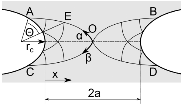
Abbildung 5.3: Gleitlinien zwischen zwei Hohlräumen; adaptiert nach [139].
