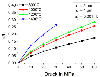
Abbildung 5.7: Modellierung der spontanen plastischen Deformation. a) Verwendung von realistischen Anfangswerten, b) die halbe Breite der Einheitszelle wird vergrößert, c) die Höhe des Hohlraums wird vermindert, d) eine Zunahme des Drucks, der Höhe der Einheitszelle, sowie der Temperatur führen zu einer Zunahme der gefügten Fläche.
