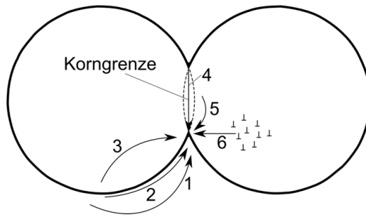
Abbildung 2.6: Schematische Darstellung der Mechanismen, die bei einem Sinterprozess zum Verschmelzen von zwei Partikeln führen. Dieses sind sowohl Verdampfung und Kondensation (1) als auch Oberflächen- (2) und Volumendiffusion (3). Zudem wirkt ein diffusionsgesteuerter Materialtransport entlang (4) und neben (5) der Korngrenze durch das Gitter. Wird eine Spannung angelegt, kann auch noch ein Materialtransport durch Versetzungskriechen erfolgen (6); adaptiert nach [90, 91].
