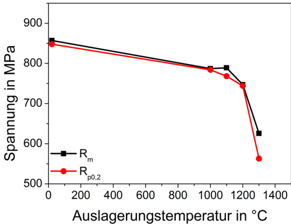
Abbildung 4.10: Zugversuche der ausgelagerten Proben. Eine deutliche Verminderung der Zugfestigkeit ist bei einer Auslagerungstemperatur von 1300 °C zu erkennen.
