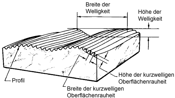
Abbildung 2.11: Schematische Darstellung der Oberflächenrauheit und der Welligkeit der Oberfläche; adaptiert nach [99].
