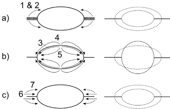
Abbildung 5.2: Schematische Darstellung der unterschiedlichen Diffusions- und Deformationsmechanismen nach Hill und Wallach [13]. Links sind die Transportwege und rechts die zeitabhängigen Formänderungen des elliptischen Hohlraums dargestellt. a) Spontane plastische Deformation (1) und Kriechen (2). b) Diffusionsmechanismen der Oberflächendiffusion (3), Volumendiffusion (4) sowie des Verdampfens und Kondensierens (5) von Material mit der Quelle an der Hohlraumoberfläche mit geringer Krümmung. c) Korngrenzen- bzw. Grenzflächendiffusion (6) und Volumendiffusion (7) mit einem Ursprung an der Grenzfläche.
