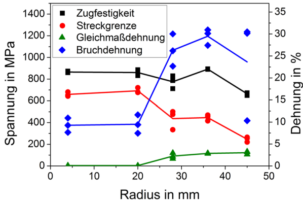
Abbildung 4.3: Charakterisierung bei Raumtemperatur von PM2000 im Anlieferungszustand. Die Zugfestigkeit, Streckgrenze, Gleichmaßdehnung und Bruchdehnung sind in Abhängigkeit des Radius aufgetragen.
