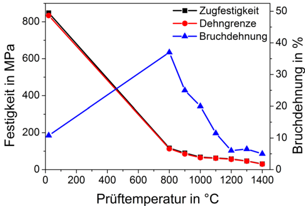
Abbildung 4.12: Die Warmzugversuche werden in einem für die Diffusionsschweißungen relevanten Temperaturbereich mit einer Dehnungsrate von 1,4 \times 10^{-7} \text{ s}^{-1} durchgeführt. Die Zugfestigkeit, Dehngrenze und Bruchdehnung nehmen mit steigender Prüftemperatur ab.
