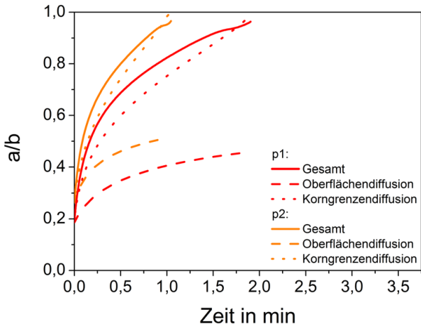
Figure 6.13: Simulation der Hohlräumschließung mit den Parametersätzen aus Tabelle 6.4. Je höher der Diffusionsschweißdruck, desto geringer ist die benötigte Diffusionsschweißzeit.
