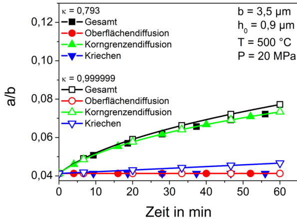
Abbildung 5.8: Simulation des Diffusionsschweißens unter Variation des Relaxationsfaktors. Der experimentell ermittelte Relaxationsfaktor \kappa = 0,793 erzeugt keinen Einfluss des Kriechmechanismus auf die Schließung des Hohlraums. Eine deutliche Vergrößerung des Relaxationsfaktors führt zu einer Beschleunigung der Verschweißung. Zur Sichtbarmachung ist ein verhältnismäßig niedriger Druck und eine niedrige Temperatur gewählt. Die Erhöhung der Temperatur führt zur schnelleren Versetzungsbewegung aber auch zu schnelleren Diffusionsprozessen. Eine Druckerhöhung fördert neben dem Kriechmechanismus die Grenzflächendiffusion, die bei sehr hohen Drücken und Temperaturen dominiert und den Einfluss des Kriechmechanismus minimiert.
