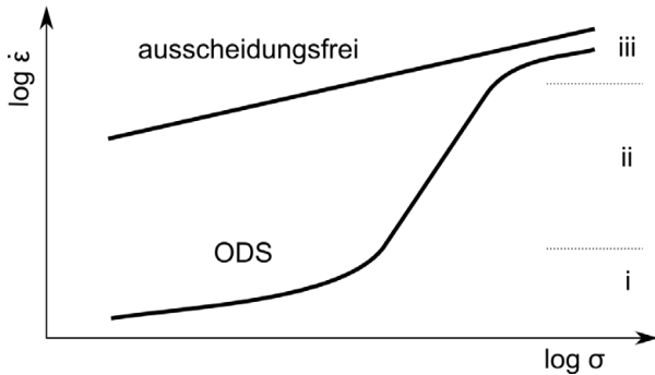
Abbildung 2.2: Schematische Darstellung der Kriechrate über der angelegten Spannung; adaptiert nach [16]
