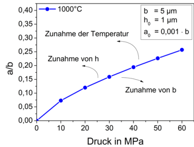
Abbildung 5.7: Modellierung der spontanen plastischen Deformation. a) Verwendung von realistischen Anfangswerten, b) die halbe Breite der Einheitszelle wird vergrößert, c) die Höhe des Hohlraums wird vermindert, d) eine Zunahme des Drucks, der Höhe der Einheitszelle, sowie der Temperatur führen zu einer Zunahme der gefügten Fläche.
