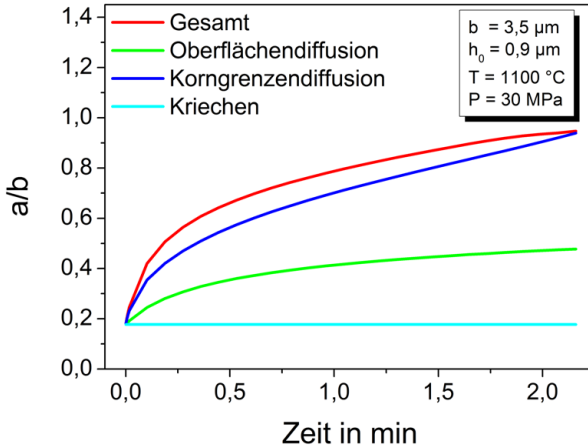
Abbildung 5.9: Modellierung der Hohlraumschließung mit allen beteiligten Mechanismen.
