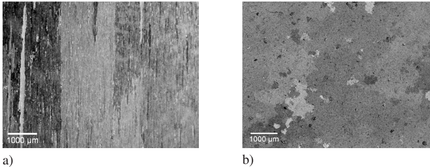
Abbildung 4.1: Lichtmikroskopische Aufnahmen von angeätztem PM2000 a) Korngefüge längs und b) quer zur Extrusionsrichtung [131].
