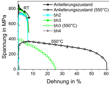
a) Zugversuche
