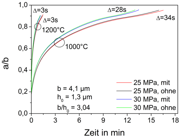
Abbildung 5.6: Einfluss der Verwendung des Labyrinthkoeffizienten auf die Modellierung des Diffusionsschweißprozesses. Der Einfluss der Oxidpartikel auf die Diffusion ist gering. \frac{a}{b} beschreibt den Anteil der bereits gefügten Fläche.
