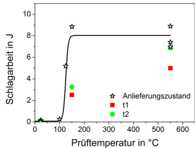
b) Kerbschlagbiegeversuche
