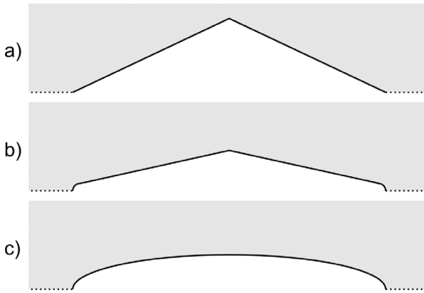
Abbildung 2.10: Schematische Darstellung der unterschiedlichen Oberflächengeometrien, mit denen der Grenzflächenhohlraum modelliert wird. a) Die Hohlräume werden durch Dreiecke beschrieben [72]. b) An der Kontaktfläche werden Viertelkreise an die Dreiecksform angefügt [101]. c) Elliptischer Querschnitt des Hohlräume [13].
