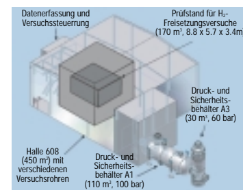
Skizze des Wasserstofftechnikums
