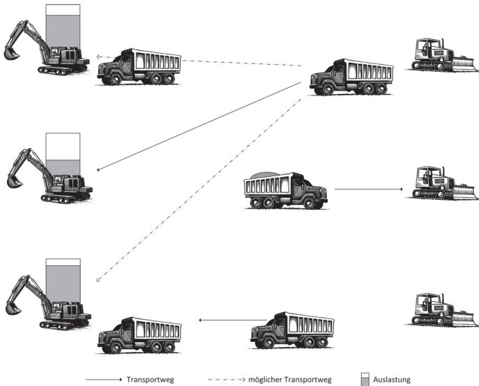
Abbildung 5.9: Kontextsensitive Zuordnung eines Dumpers zu einem Bagger
