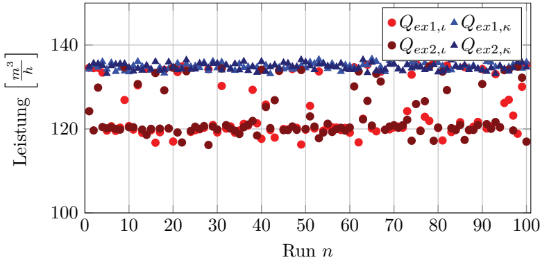
Abbildung 6.9: Simulation Baustelle I (zusätzlicher Dumper): Leistung
