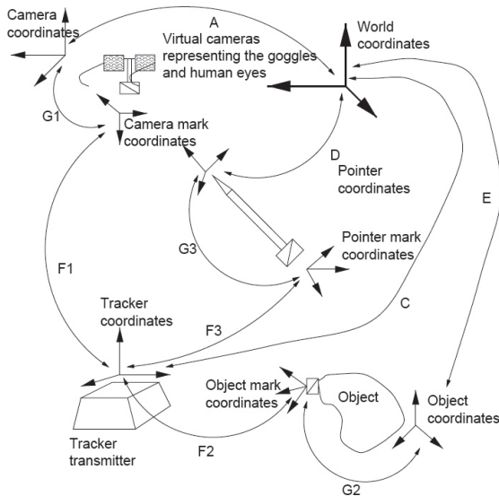
Abbildung 2.12: Koordinatensysteme und ihre Verhältnisse zueinander [275]
