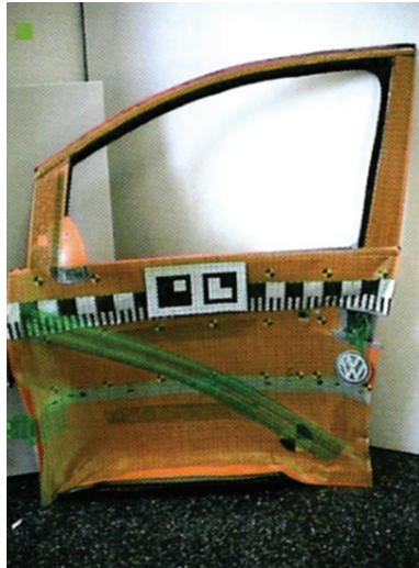
Abbildung A.6: ARVIKA: Augmentierte, gecrashte Fahrzeugtür mit Simulationsdaten [131]
