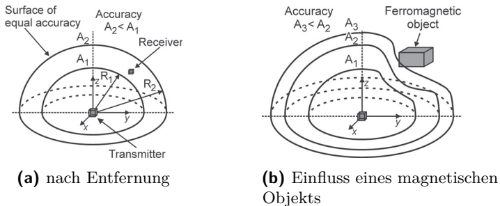
Abbildung 2.10: Genauigkeit magnetischer Tracker [68]
