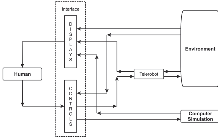
Abbildung 2.14: Schematische Darstellung eines AR-Systems [109]
