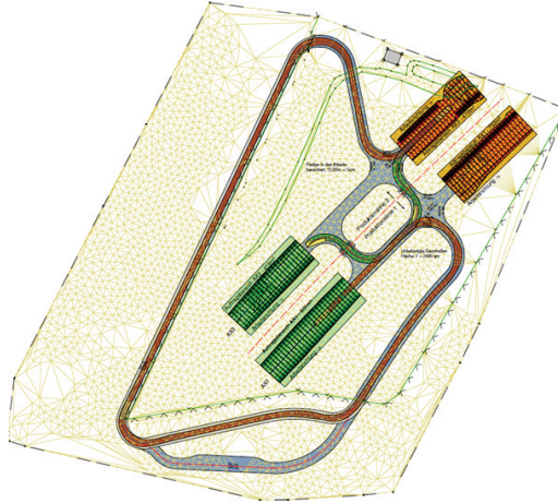
Abbildung 5.21: Plan Walldorf [56]
