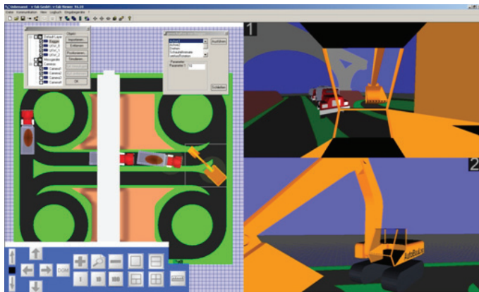
Abbildung 6.2: Modellhafte Implementierung des Leitstands [225]
