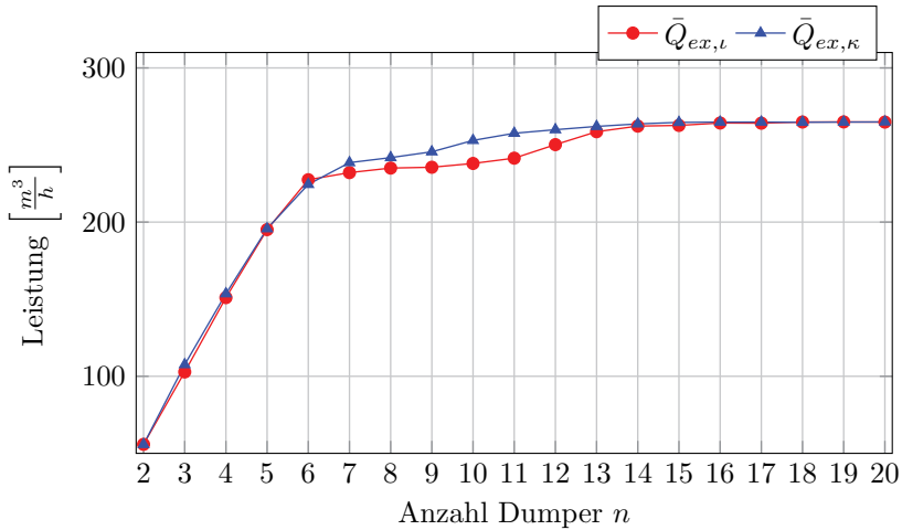
Abbildung 6.11: Simulation Baustelle I: Leistung in Abhängigkeit der Dumper-Anzahl
