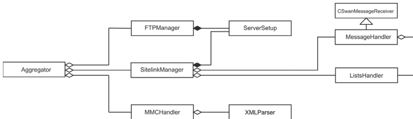
Abbildung C.14: Klassenhierarchie Aggregator
