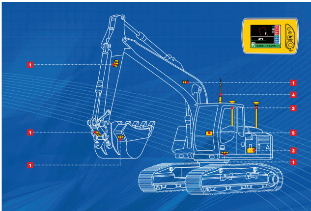
Abbildung 5.3: 3D-Maschinensteuerung für Bagger (nach [410])
