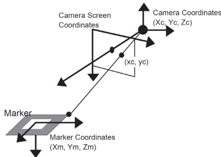
Abbildung C.2: Beziehung zwischen Kamera- und Marker-Koordinatensystem [217]
