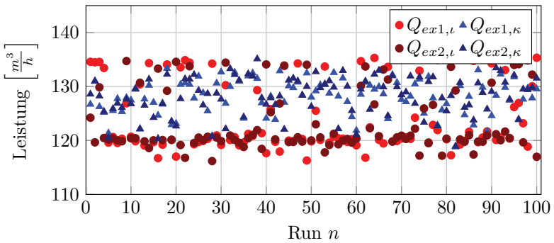
Abbildung A.17: Simulation Baustelle I: Leistung
