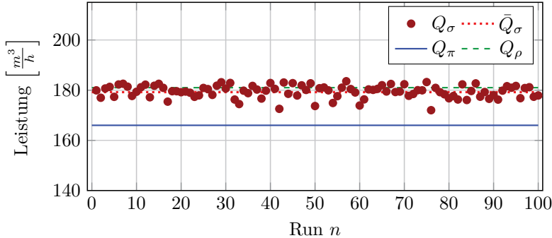
Abbildung 5.20: Simulationsergebnisse zur Leistungsberechnung der Baumaßnahme A
