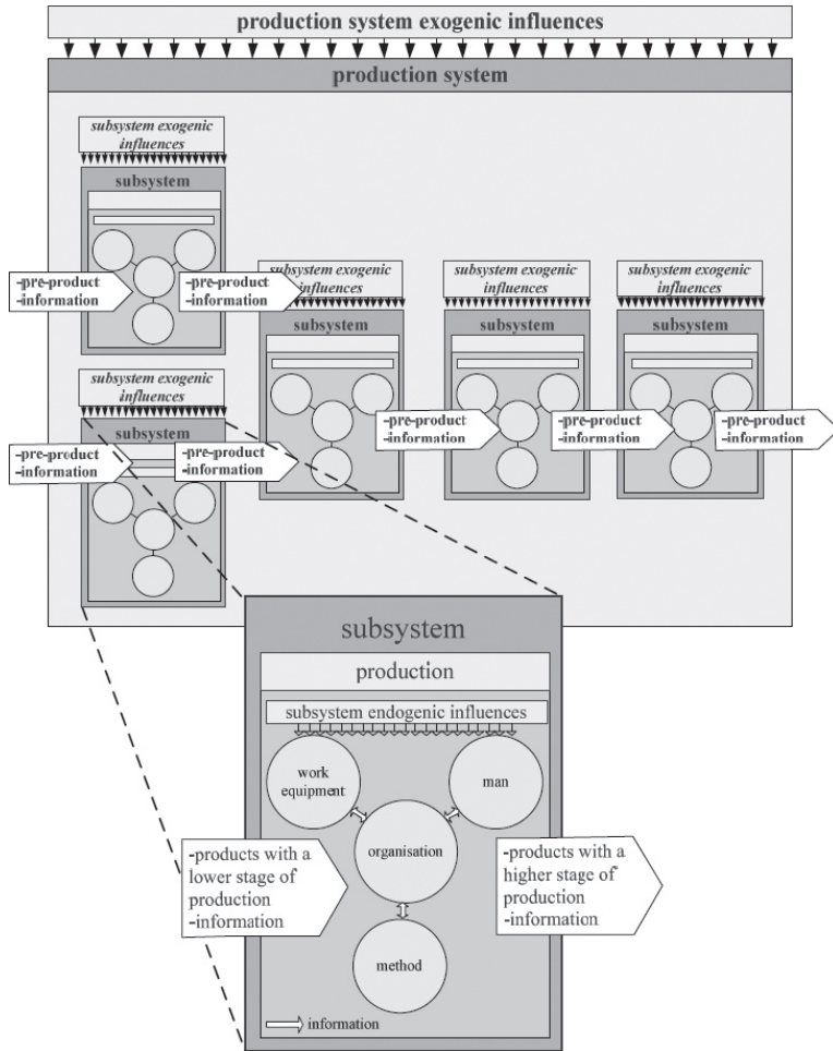
Abbildung 3.1: Aufbau eines Produktionssystems [223]
