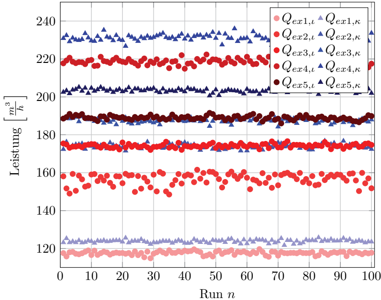
Abbildung 6.10: Simulation Baustelle II: Leistung
