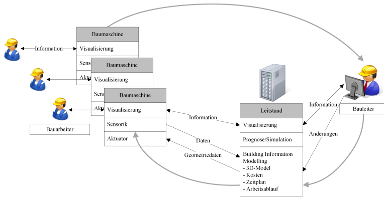
Abbildung 5.5: Leitstandarchitektur
