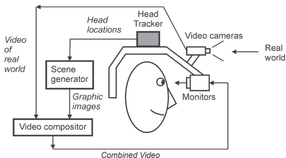
Abbildung 2.19: Konzept „Video See-Through“ [17]
