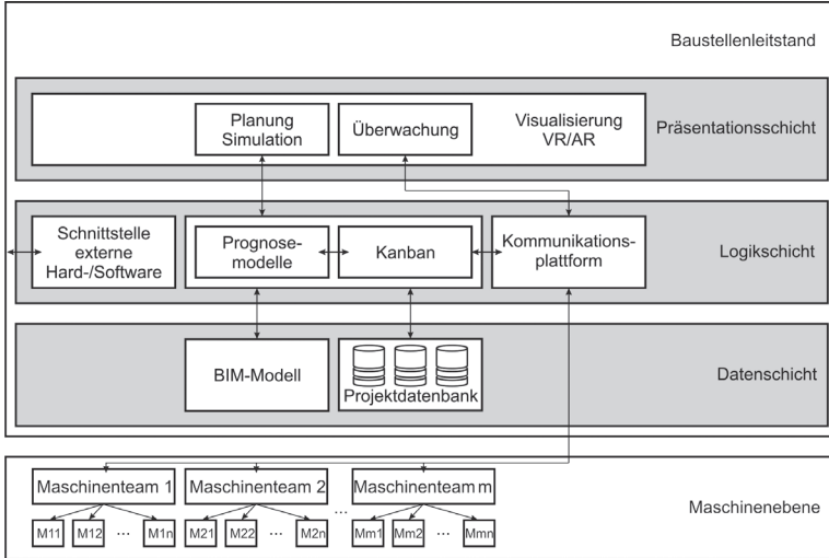
Abbildung 5.6: Interner Aufbau des VR-Leitstands
