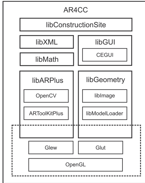
Abbildung 5.12: AR4CC-Architektur
