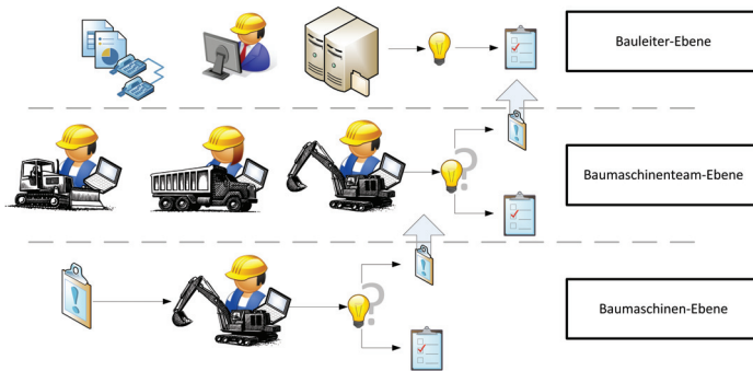
Abbildung 5.11: Ebenenkonzept des Leitstands
