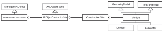
Abbildung C.9: Klassenhierarchie Baustelle
