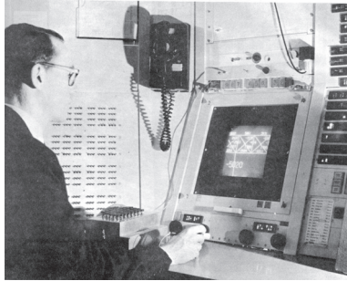
Abbildung A.2: Benutzung des Sketchpads [388]
