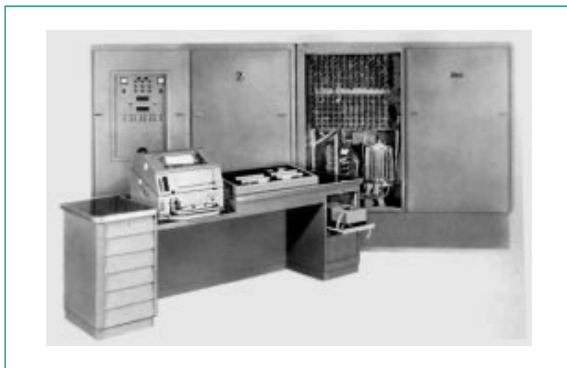
Abb. 3: Röhrenrechner Z22 von 1959.
