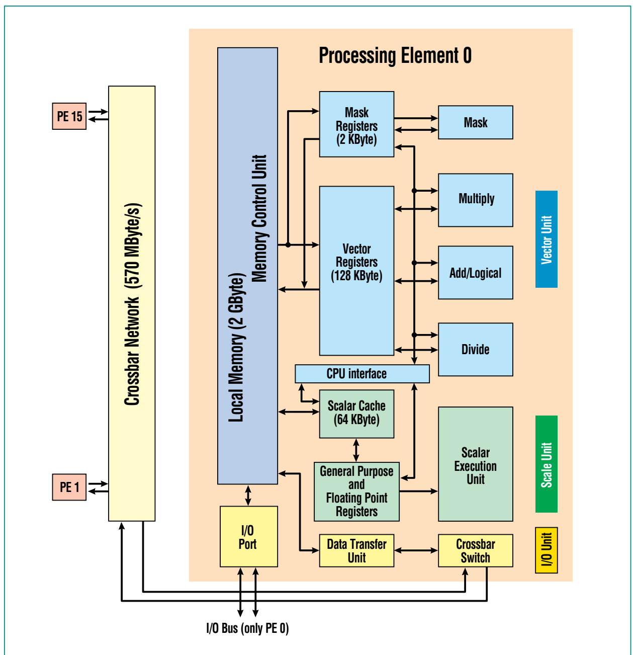
Abb. 4: Schaltbild des VPP300.
