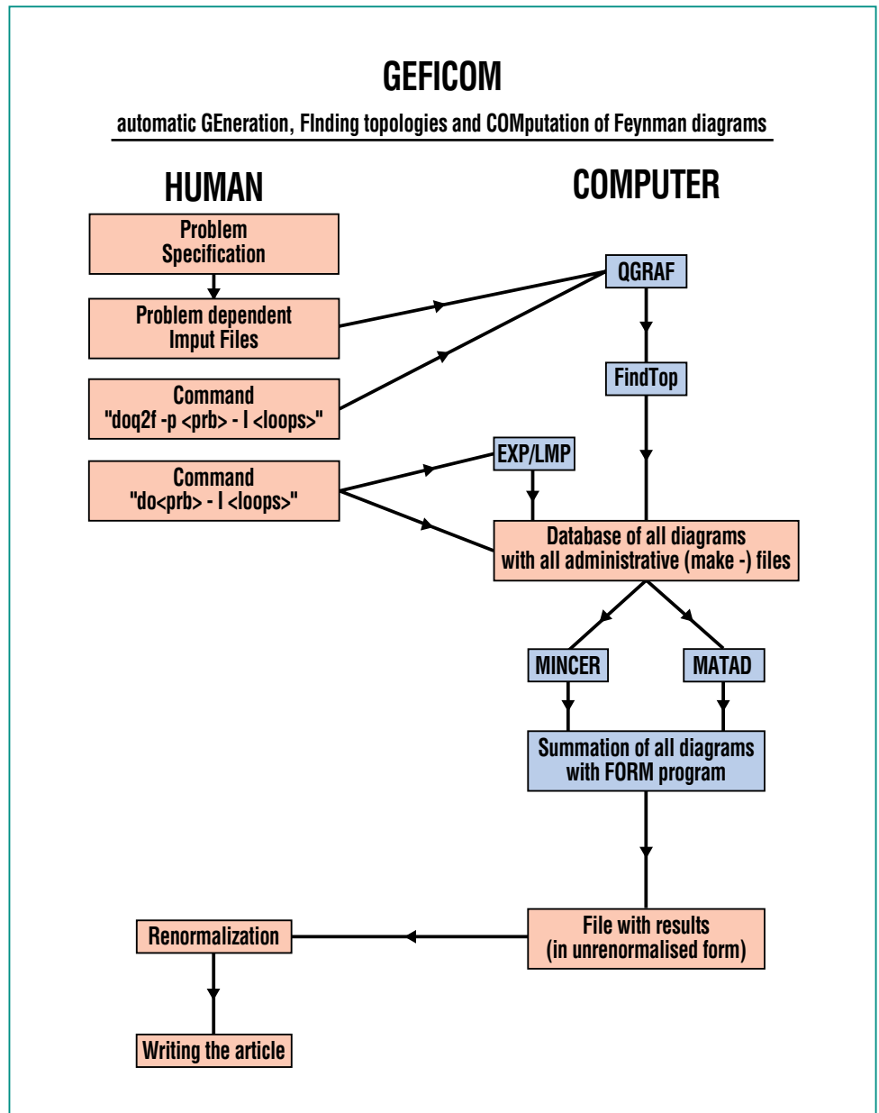
Abb. 2: Flussdiagramm von GEFICOM.
