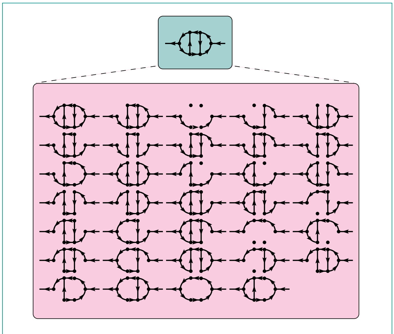
Abb. 3: Diagrammatische Darstellung der asymptotischen Entwicklung des in der ersten Zeile dargestellten Diagramms für den Fall, dass der äußere Impuls viel größer ist als die Masse der virtuellen Teilchen.
