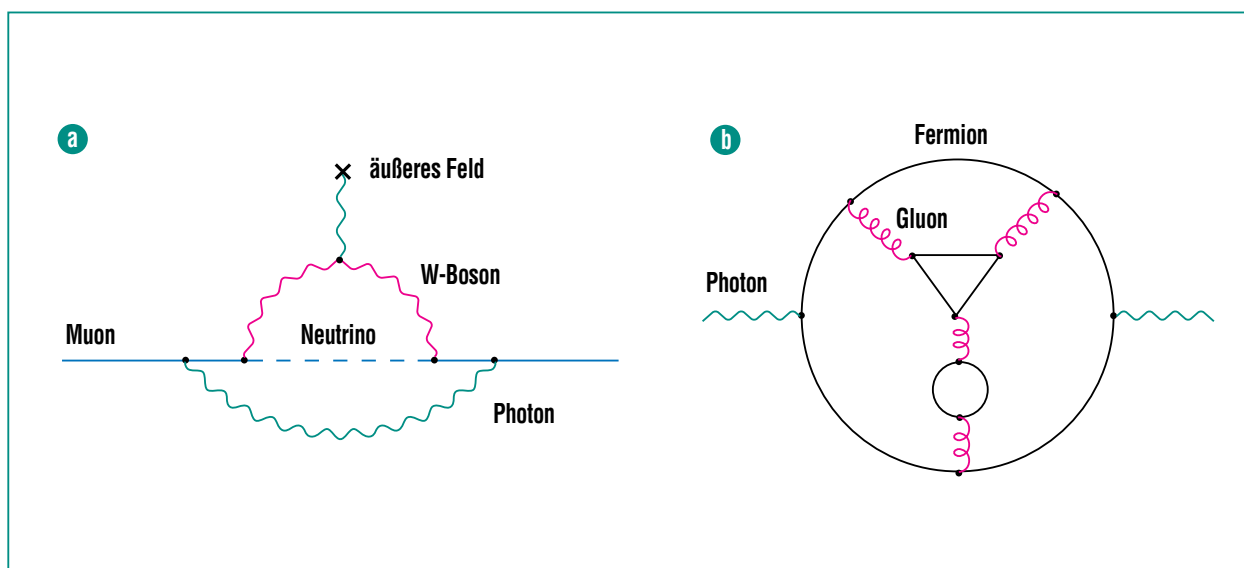
Abb. 1: Beispiele für kurzzeitige Teilchen-Antiteilchen-Erzeugung und -Vernichtung in der Teilchenphysik: (a) Feynmandiagramm, das zum anomalen magnetischen Moment des Muons in Zweischleifen-Näherung beiträgt; (b) Beitrag zur Vakuumpolarisation in Fünfschleifen-Näherung der Quantenchromodynamik. Gluonen sind die Vermittler der starken Wechselwirkung.
