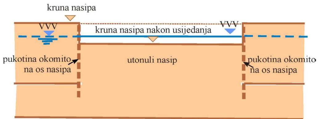
Slika 8.13 Usjedanje nasipa
