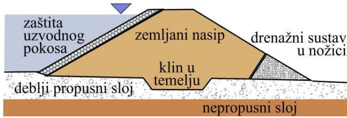
Slika 6.19 Homogeni nasip na debljoj propusnoj podlozi s klinom u temelju, oblogom uzvodnog pokosa i izvodnim drenom
