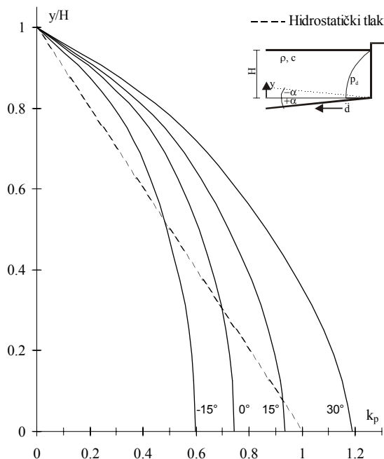
Crtež 3.P4 – Hidrodinamički tlakovi na krutu pregradu u ovisnosti o nagibu podloge
