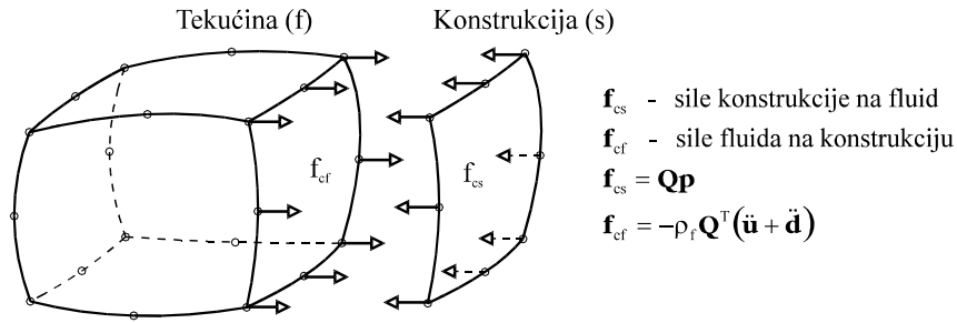
Crtež 4.2 - Ploha međudjelovanja tekućina-konstrukcija
