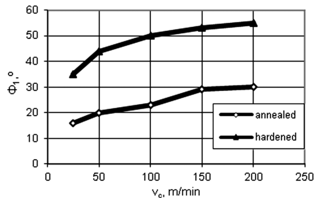
Figure 10: Influence of cutting speed on shear angle Slika 10: Vpliv hitrosti rezanja na strižni kot
